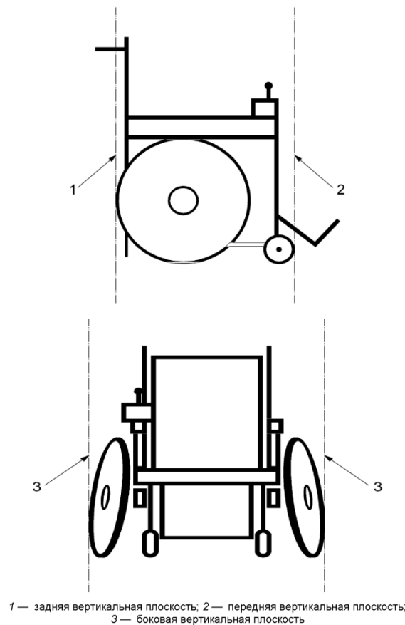
Рисунок 1 — Базовые плоскости
