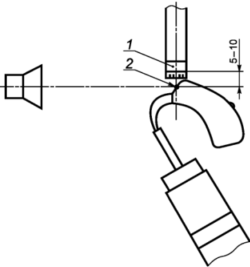
1 — контрольный микрофон; 2 — акустический вход СА
