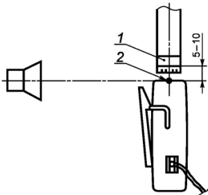
1 — контрольный микрофон; 2 — акустический вход СА
