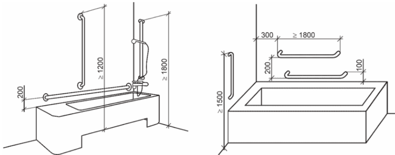
Рисунок 26 - Примеры размещения поручней у ванны
