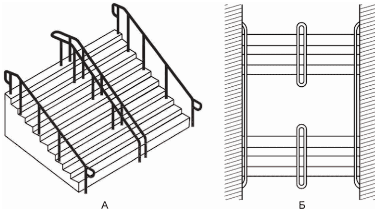
Рисунок 8 - Разделительные поручни на широких лестницах
