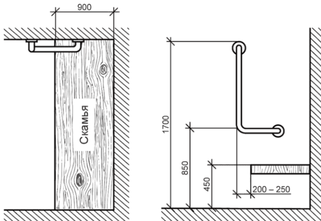
Рисунок 33 - Поручни в доступной примерочной кабине
