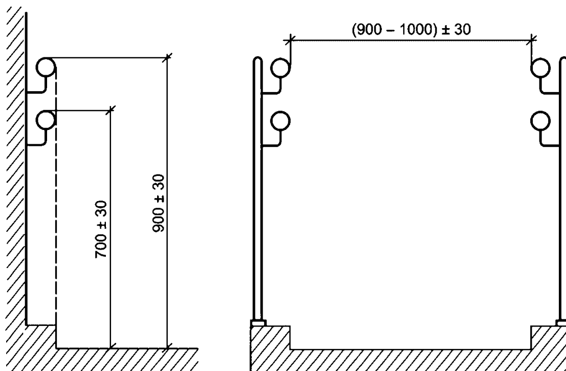
Рисунок 6 - Высота поручней и расстояние между поручнями
