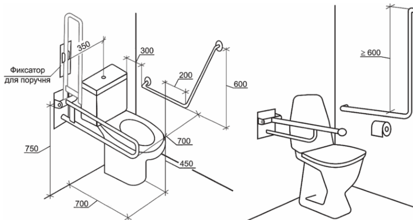
Рисунок 22 - Примеры установки комбинированных настенных поручней у унитаза
