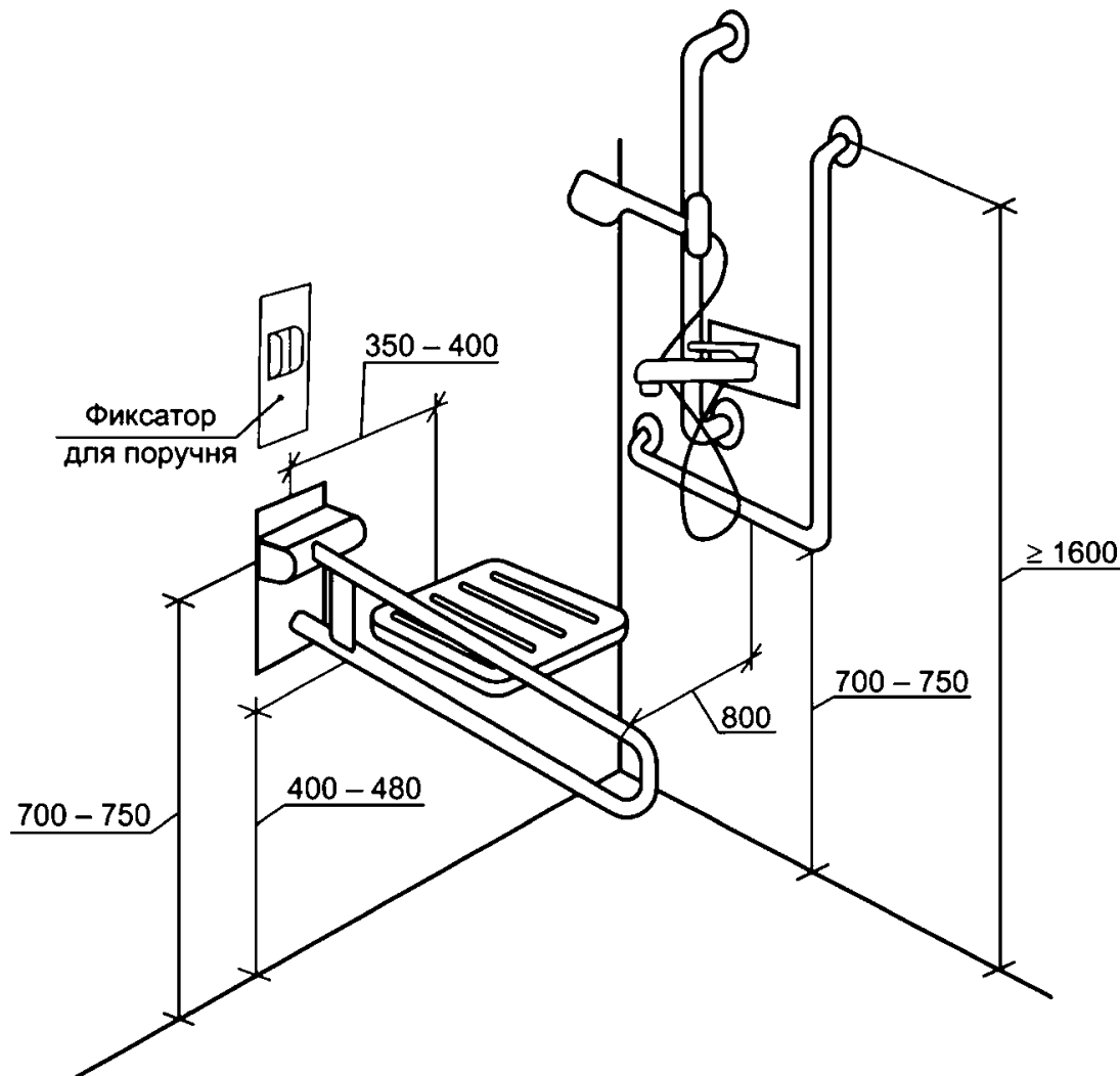
Рисунок 27 - Расположение опорных поручней в доступной душевой кабине
