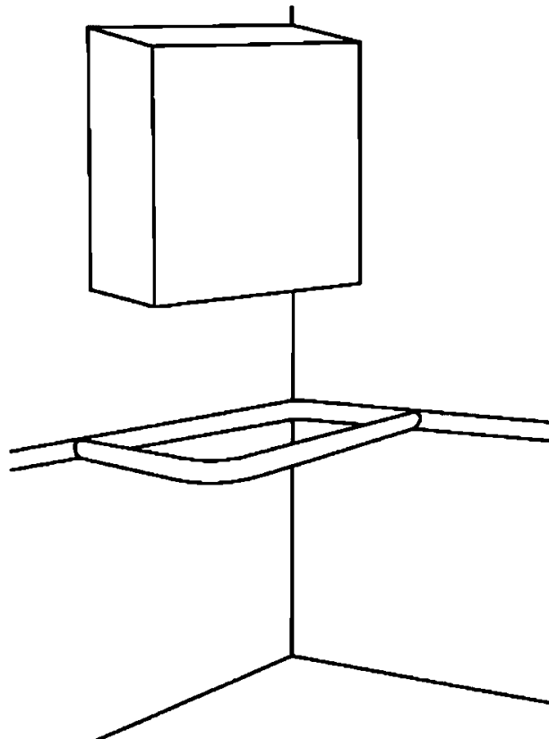
Рисунок 16 - Размещение поручней под нависающими препятствиями
