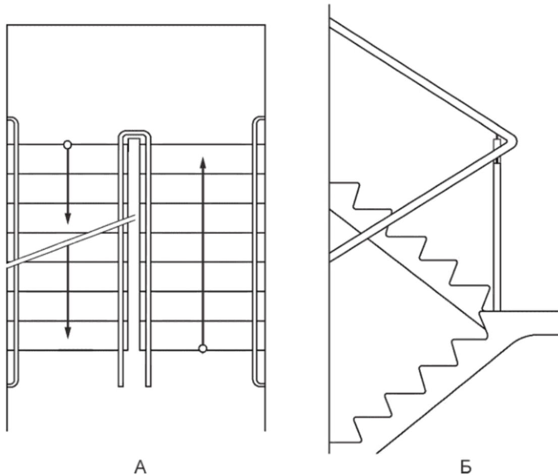
Рисунок 10 - Непрерывность внутреннего поручня многомаршевой лестницы
