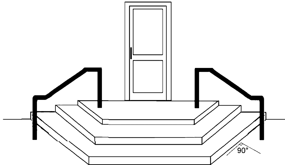
Рисунок 9 - Поручни на трехсторонних лестницах
