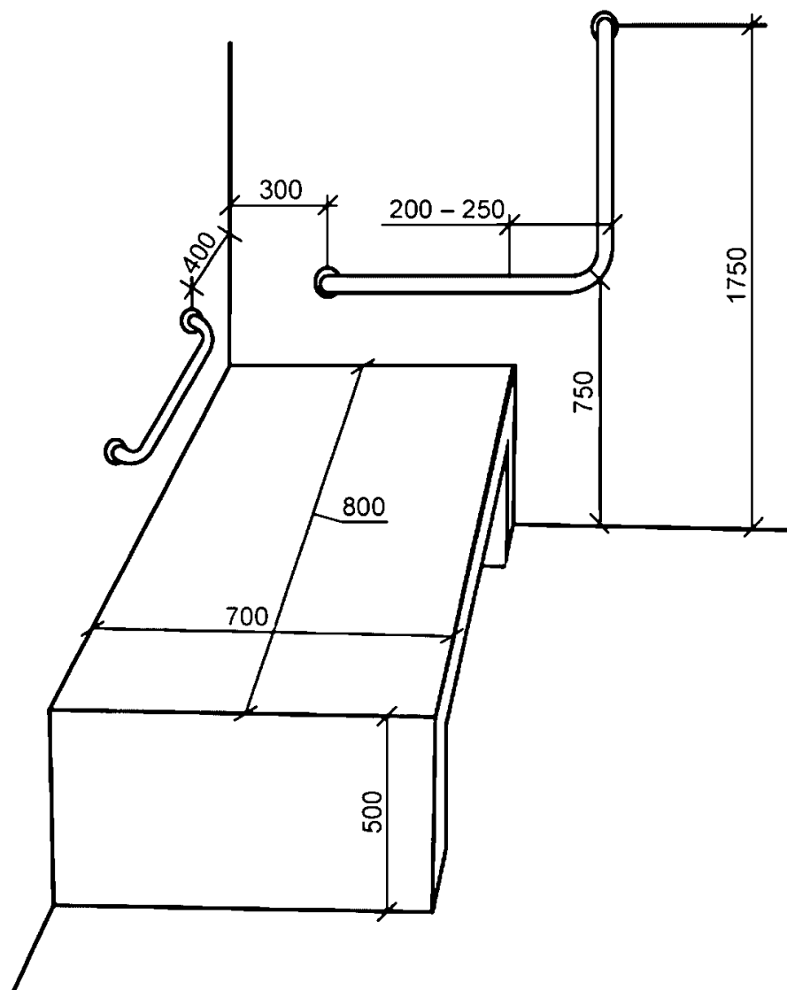
Рисунок 32 - Поручни у скамьи для переодевания
