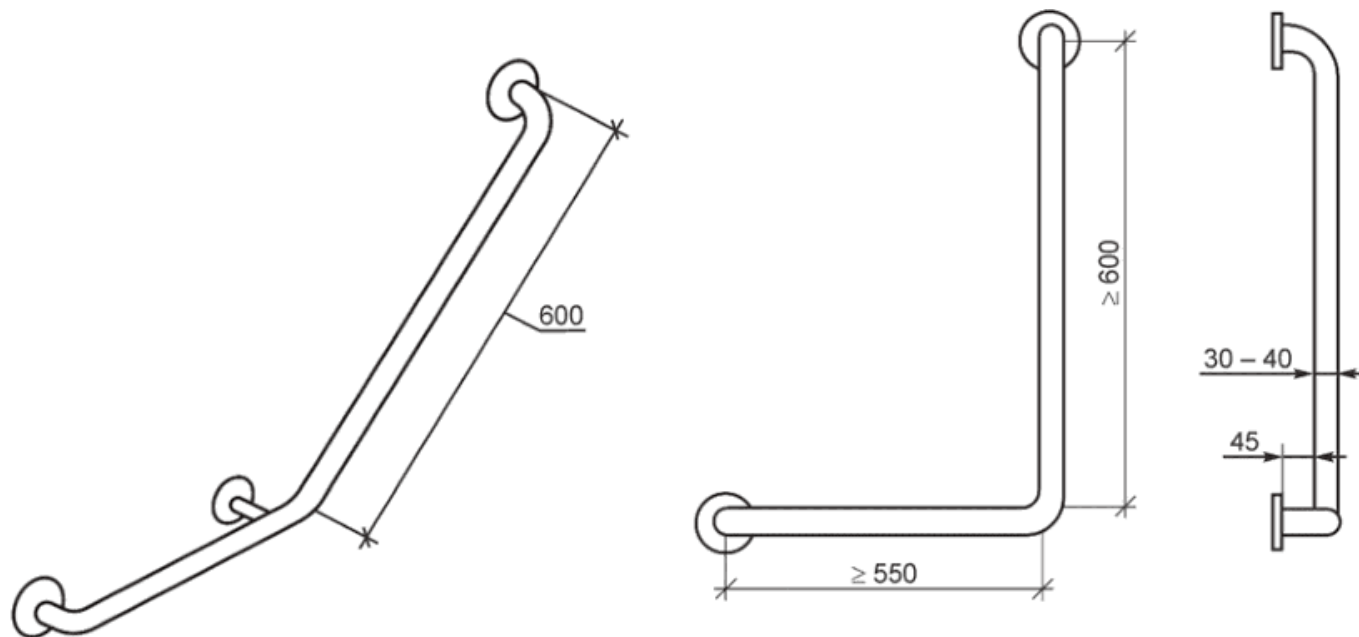
Рисунок 23 - Примеры конструкции комбинированных поручней
