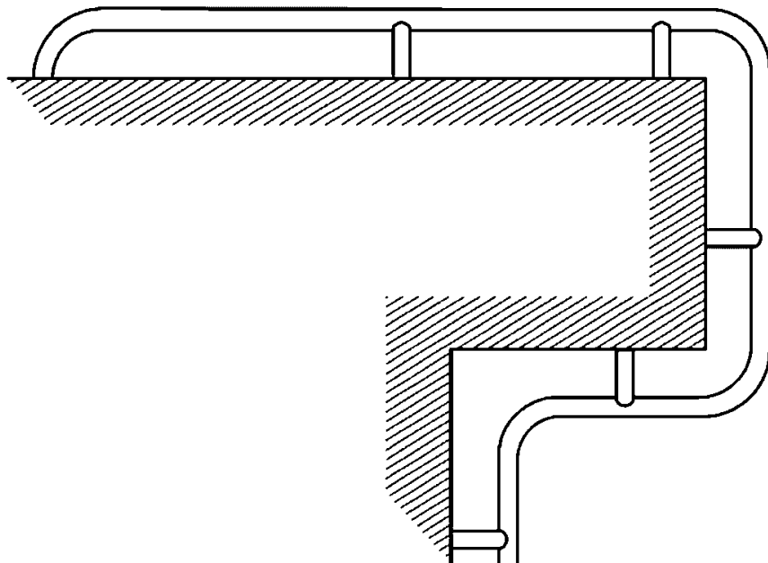
Рисунок 15 - Поручни на поворотах путей движения
