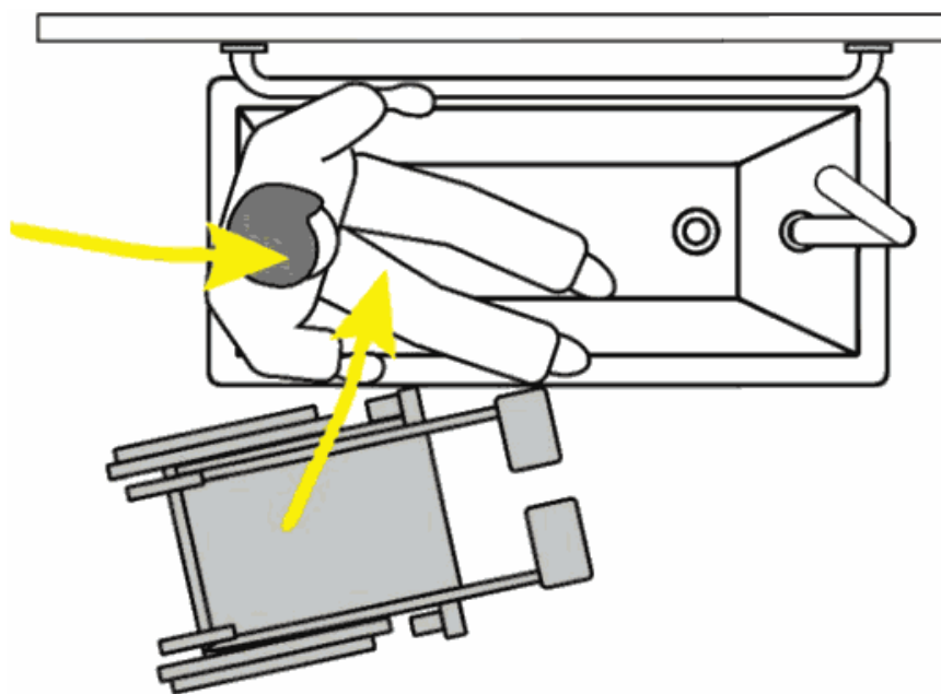
Рисунок А.20 - Варианты пересадки из кресла-коляски в ванну
