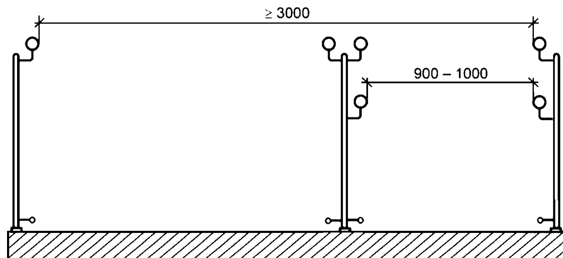
Рисунок 7 - Расположение поручней на пандусе шириной более 3 м
