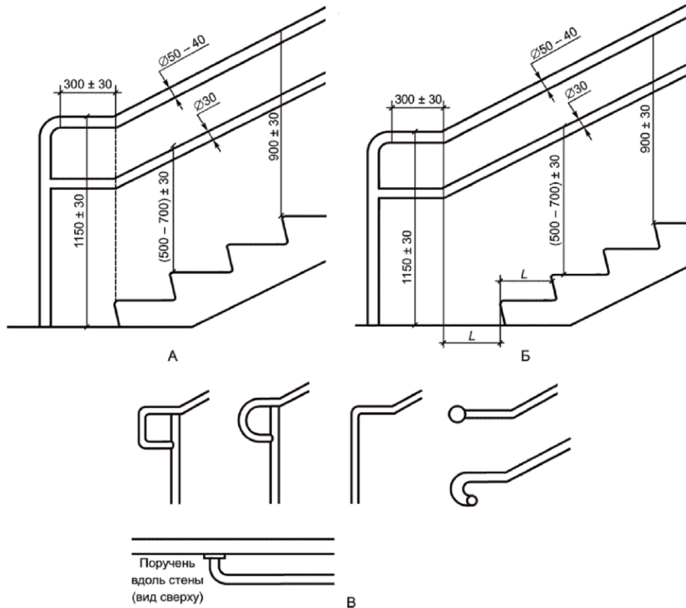
Рисунок 12 - Завершения поручней на лестнице
