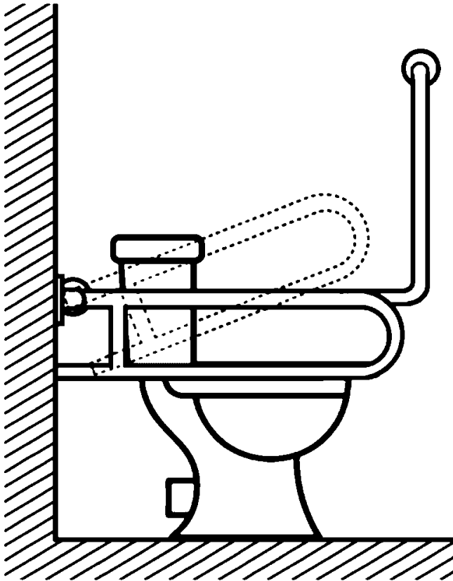
Рисунок 30 - Поручни у детского унитаза
