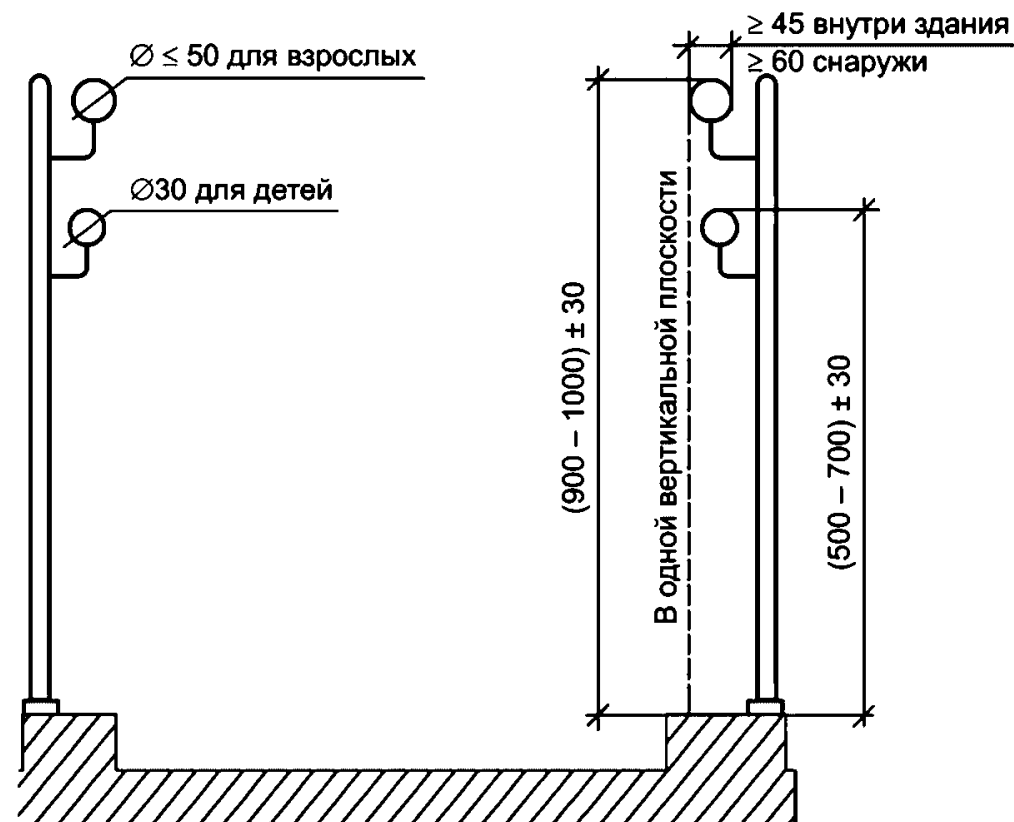
Рисунок 14 - Поручни на путях движения
