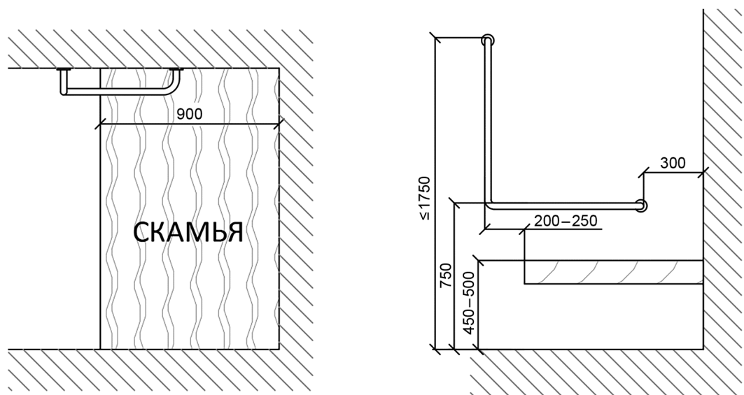
Рисунок 39 — Поручни в доступной примерочной кабине
