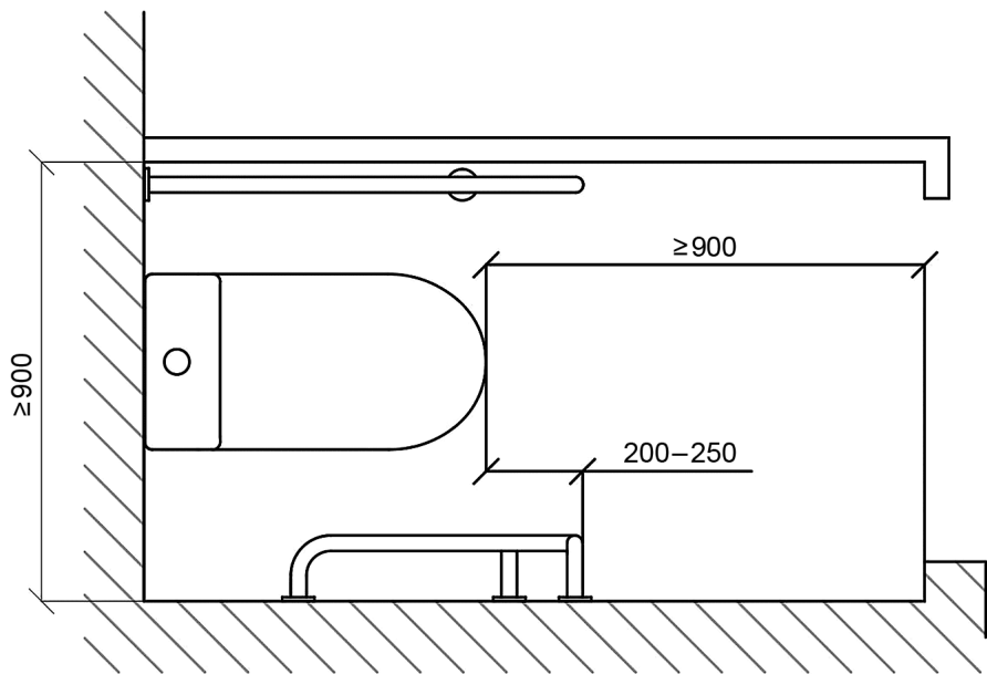
Рисунок 30 — Комбинированный поручень в адаптированной кабине уборной в блоке мужских и женских санитарно-бытовых помещений
