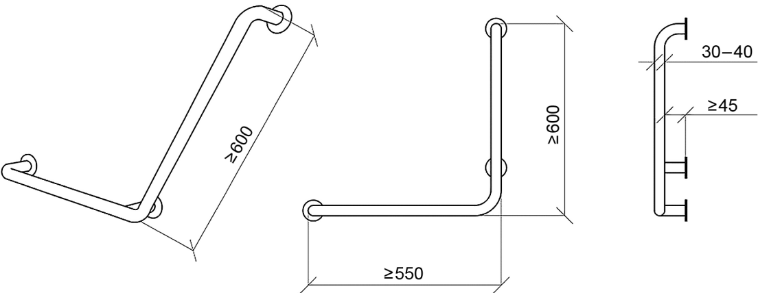
Рисунок 29 — Примеры конструкции комбинированных поручней
