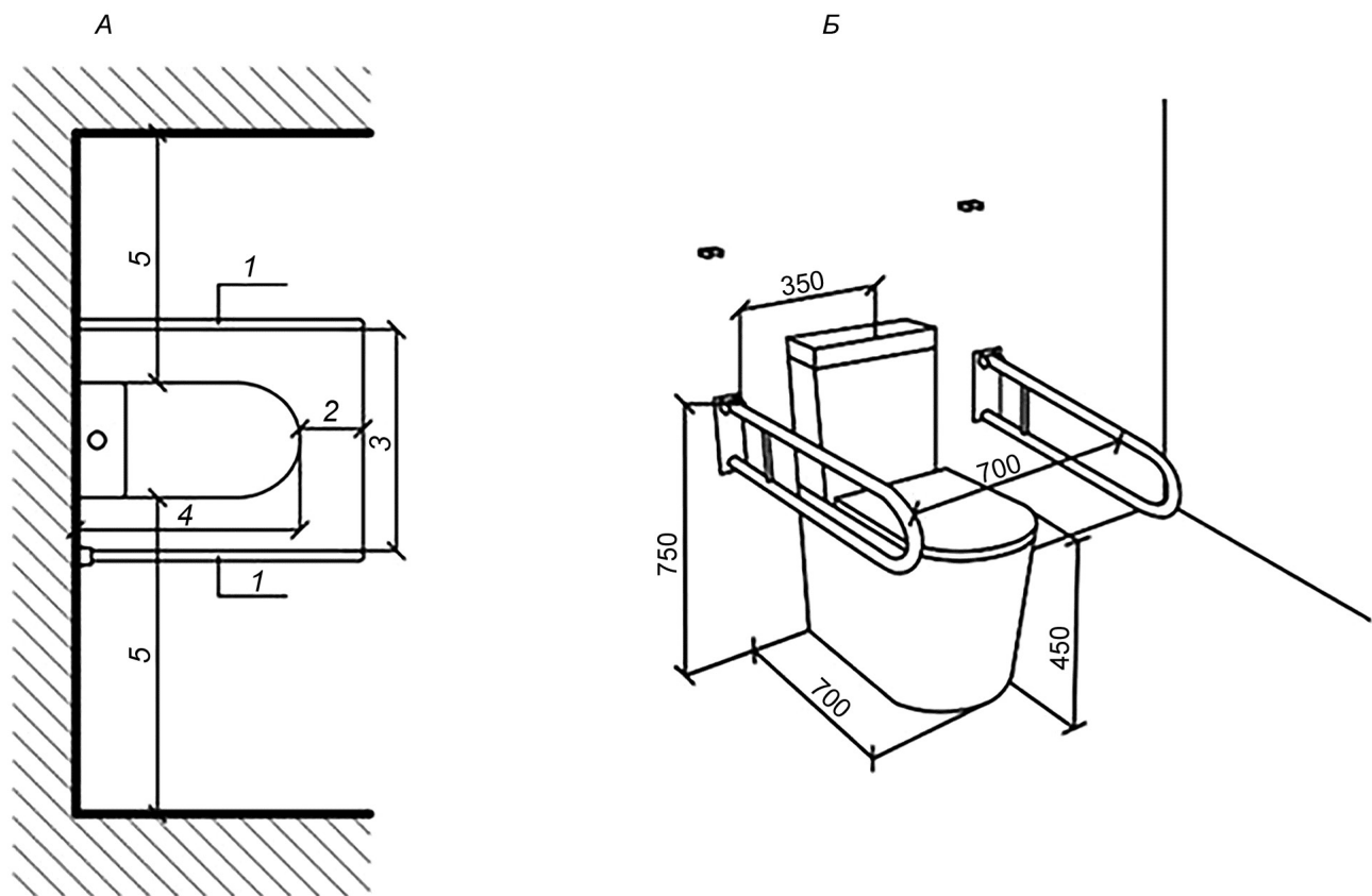
А — вид сверху; Б — объемное представление; 1 — откидной поручень; 2 — вынос поручня — не менее 150 мм; 3 — расстояние между поручнями от 700 до 750 мм; 4 — длина унитаза 700 мм; 5 — ширина зоны для размещения кресла-коляски \geq 800 мм (при реконструкции \geq 750 )
