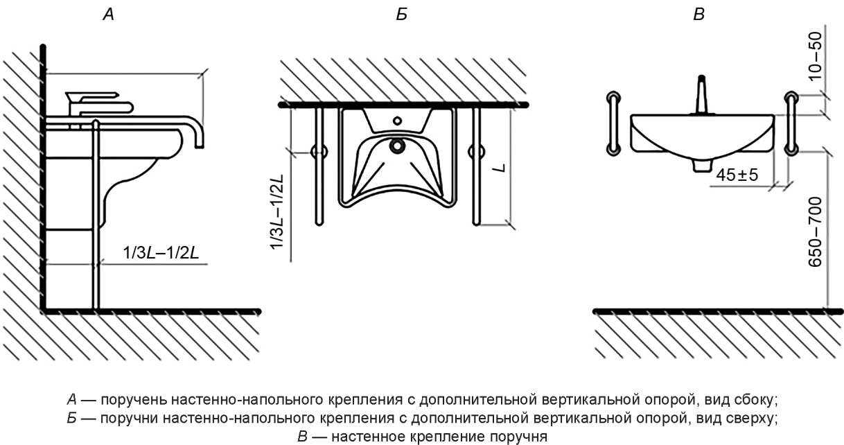
Рисунок 34 — Расположение поручней в универсальных кабинках в санитарно-бытовых помещениях у раковины
