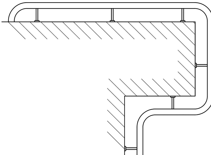
Рисунок 18 — Пример поручней на поворотах путей движения
