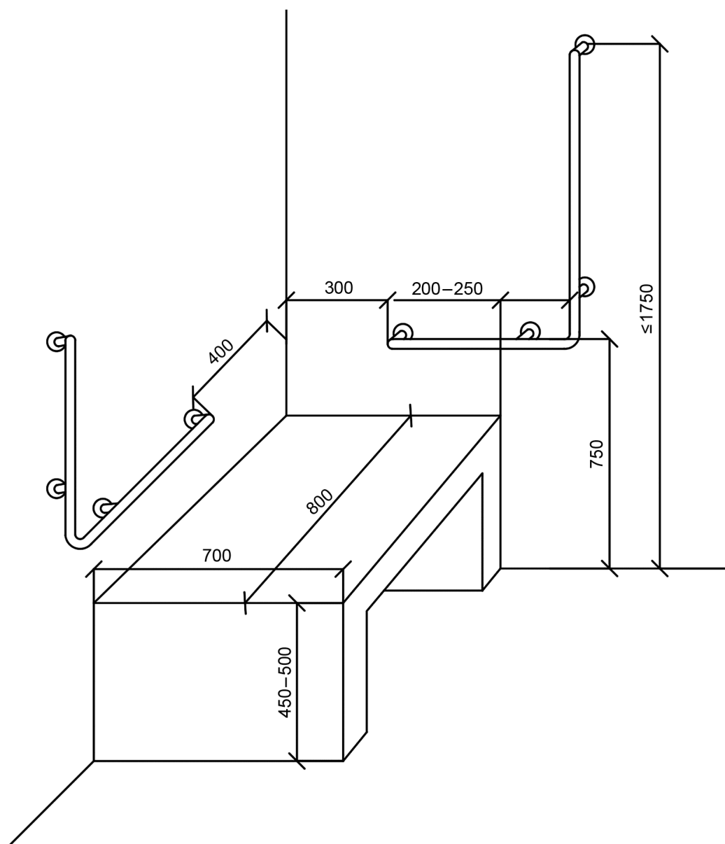
Рисунок 38 — Поручни у скамьи для переодевания
