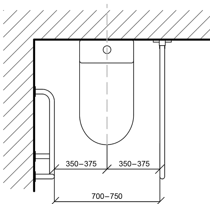
Рисунок 22 — Расстояние между поручнями у унитаза
