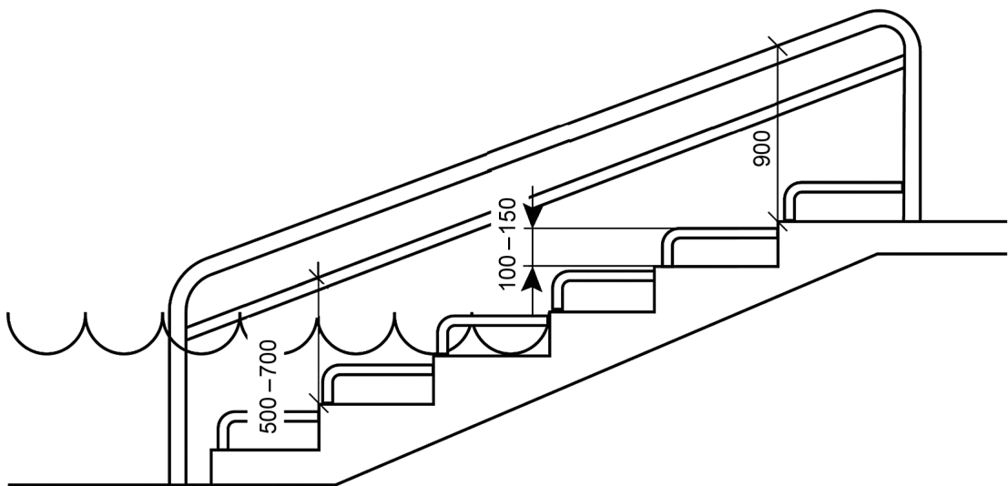
Рисунок 37 — Поручни на пологой лестнице в бассейн
