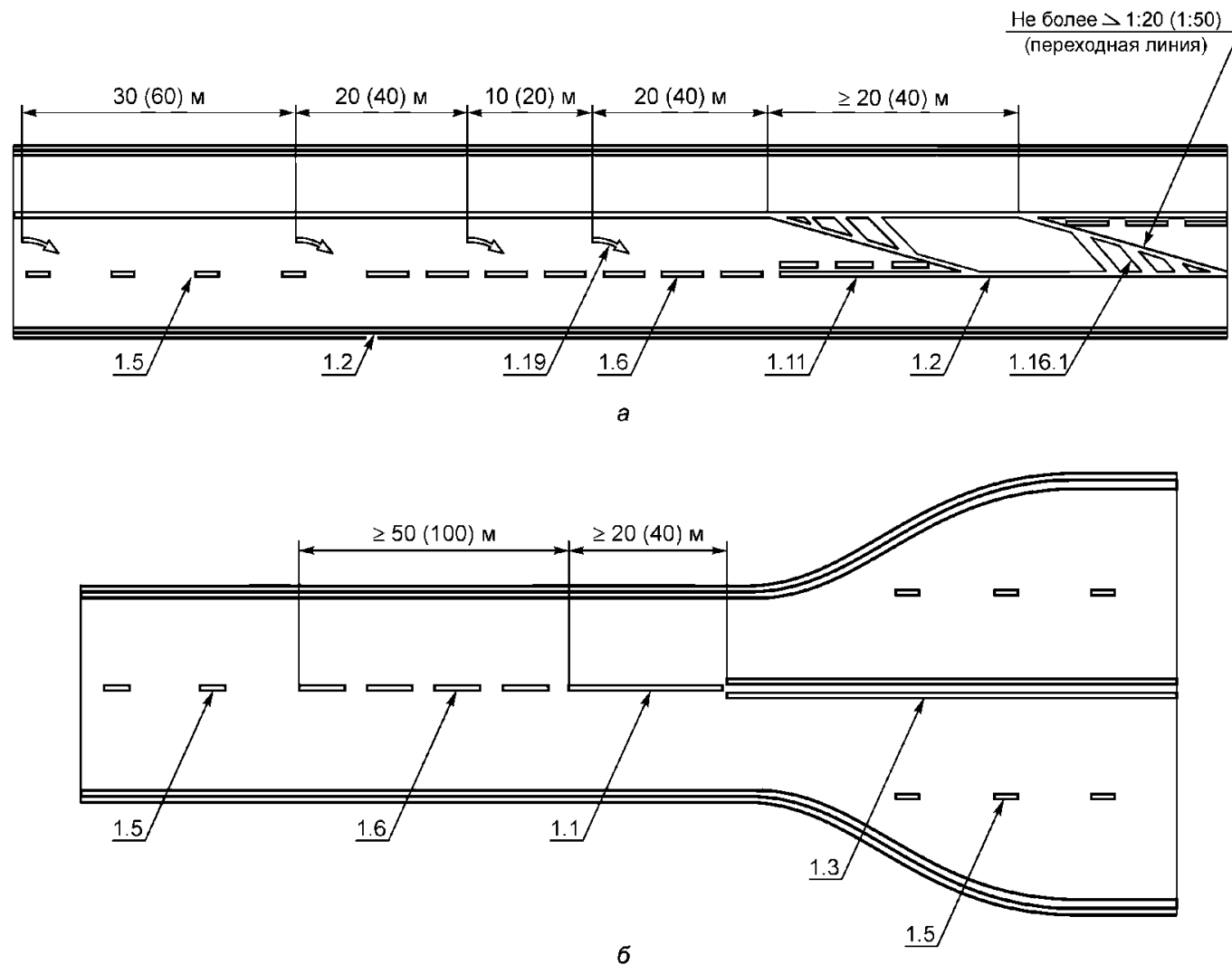
а - пример нанесения разметки при уменьшении количества полос; б - пример нанесения разметки при увеличении количества полос
