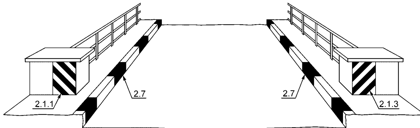
Рисунок В.23 - Пример нанесения разметки 2.1.1, 2.1.3 и 2.7
