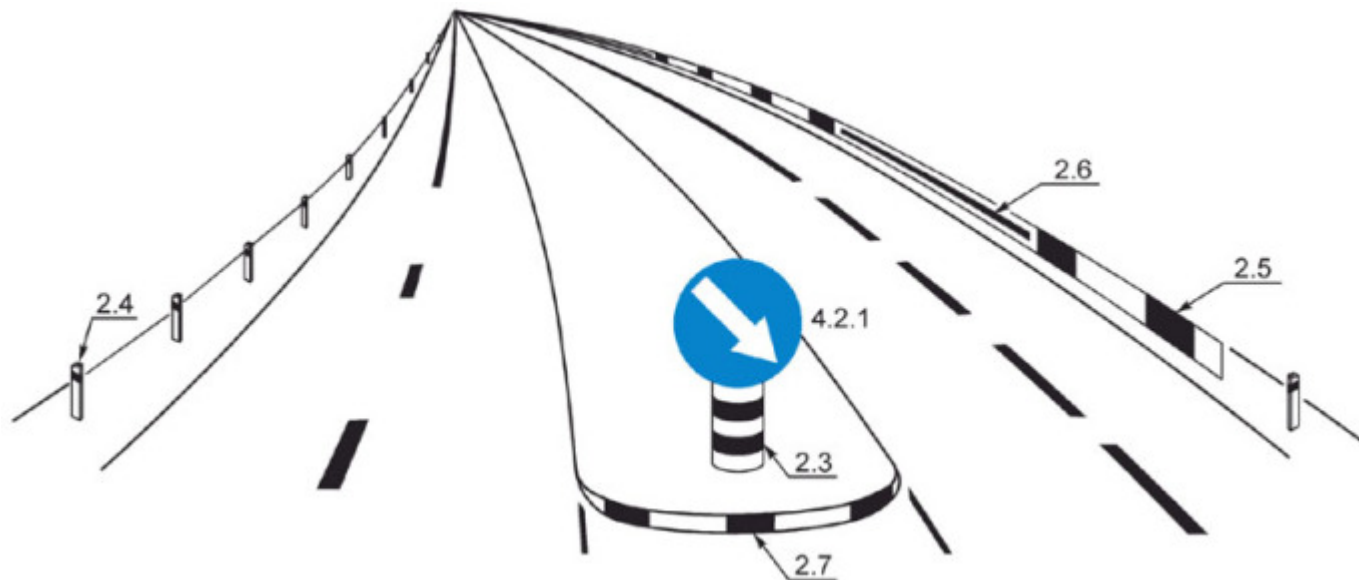
Рисунок В.24 - Пример нанесения разметки 2.3 - 2.7
