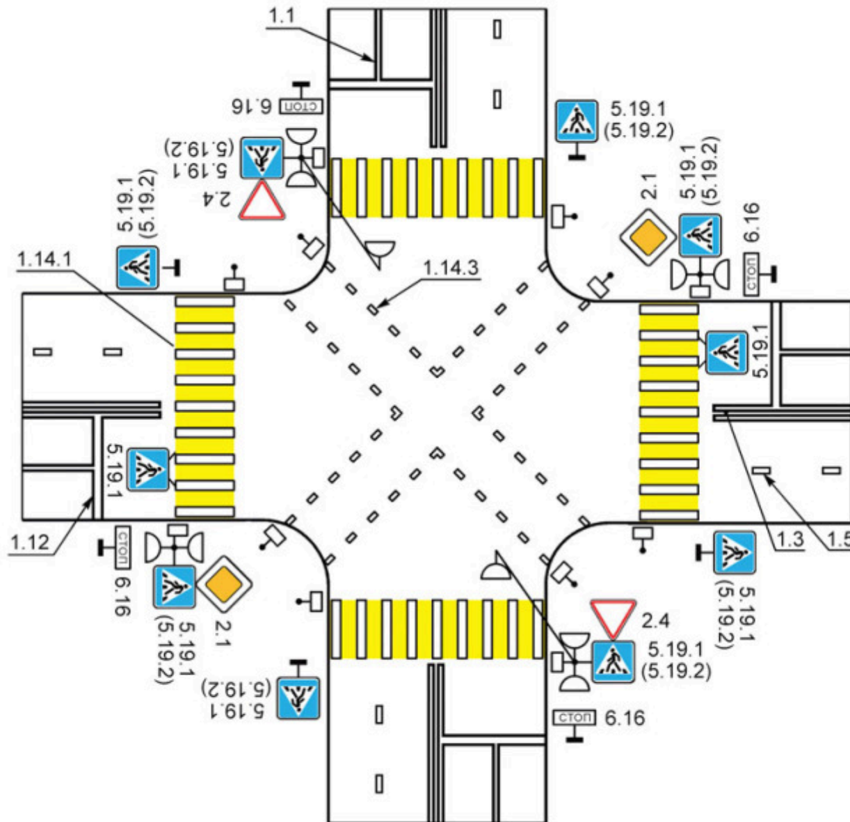
Рисунок В.19 - Пример нанесения диагонального пешеходного перехода
