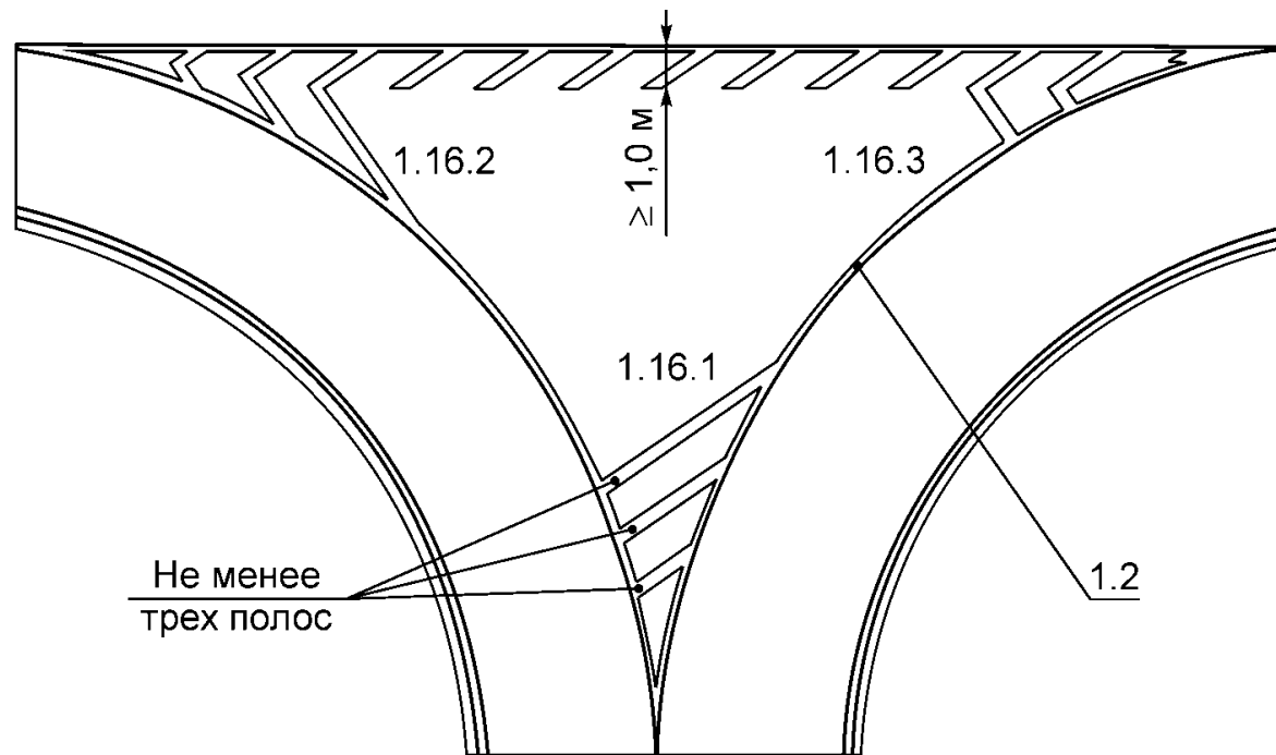
Рисунок В.12 - Пример нанесения разметки 1.16.1 - 1.16.3
