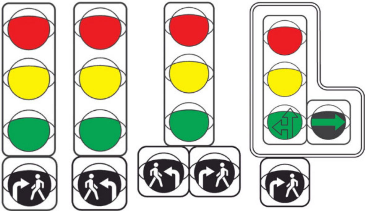
Размещение и применение ИС.п при возможном пересечении поворачивающих
