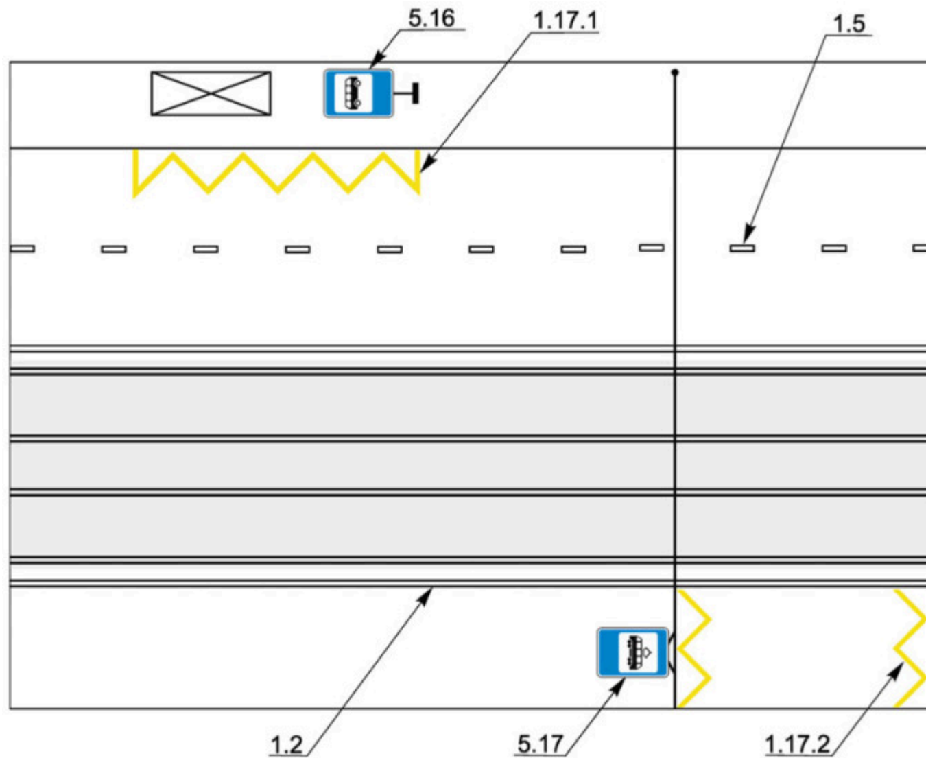
Рисунок В.15 - Пример нанесения разметки 1.17.1 и 1.17.2
