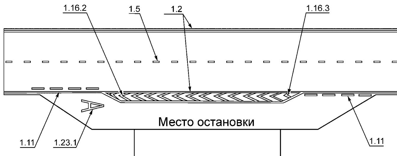
Рисунок В.13 - Пример нанесения разметки в местах организованной парковки транспортных средств
