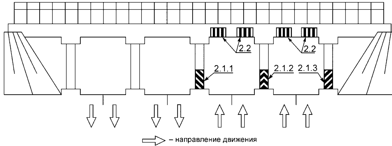
Рисунок В.22 - Пример нанесения разметки 2.1 и 2.2
