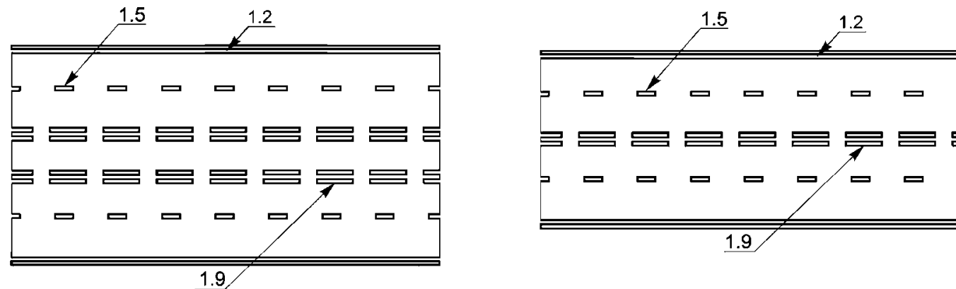
Рисунок В.17 - Примеры нанесения разметки 1.9
