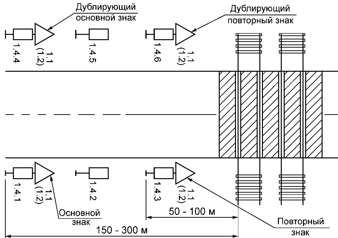
Рисунок В.3 - Размещение знаков 1.4.1 - 1.4.6
