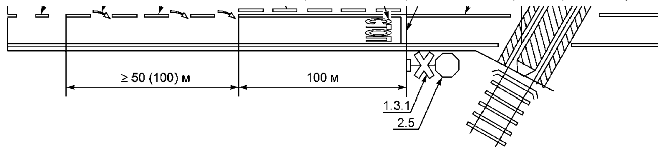
Рисунок В.18 - Примеры разметки участка дороги на подъезде к железнодорожному переезду
