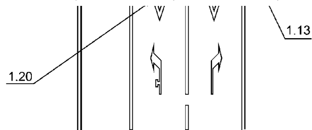
Рисунок В.10 - Пример нанесения разметки канализированного пересечения
