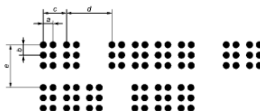
Рисунок 2 — Схема размеров рельефно-точечного шрифта Брайля
