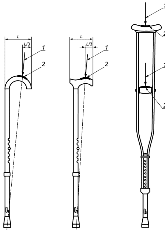
Рисунок 3 — Испытание изделий на прочность
