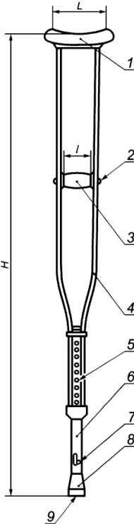
Рисунок 2 — Пример подмышечного костыля
