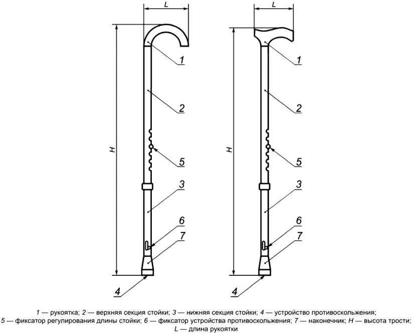
Рисунок 1 — Примеры опорных тростей
