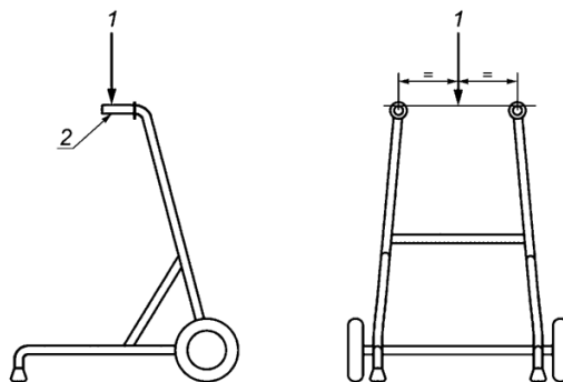
1 — нагрузка; 2 — задняя контрольная точка рукоятки
