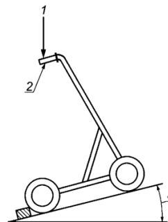
1 — нагрузка; 2 — задняя контрольная точка рукоятки; 3 — угол наклона Рисунок 8 — Схема нагружения при испытании на заднюю устойчивость
