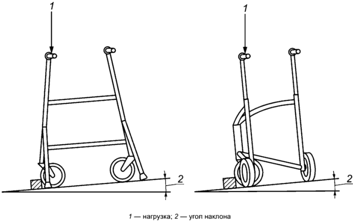
Рисунок 9 — Схема нагружения при испытании на боковую устойчивость
