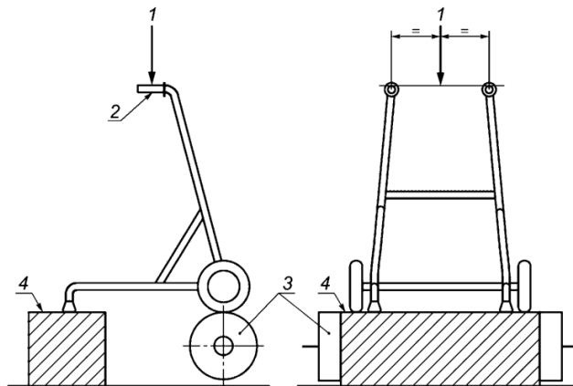
Рисунок 11 — Пример испытания на усталостную прочность для ходунков с двумя колесиками и двумя наконечниками
