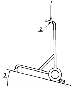
1 — нагрузка; 2 — передняя контрольная точка рукоятки; 3 — угол наклона Рисунок 7 — Схема нагружения при испытании на переднюю устойчивость
