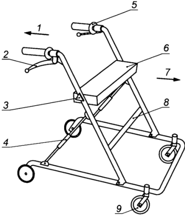
1 — направление назад; 2 — ручья тормоза; 3 — механизм регулирования высоты; 4 — механизм складывания; 5 — ручьяткя/ручка; 6 — сиденье для отдыха; 7 — направление вперед; 8 — растяжка; 9 — колесики
