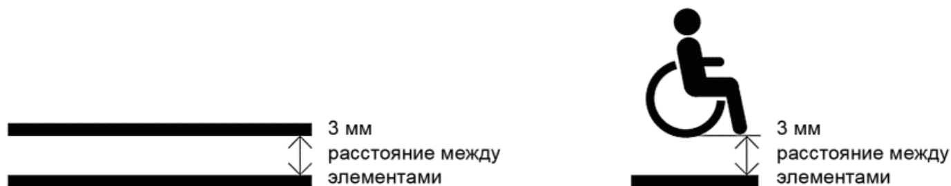
Рисунок 15 - Минимальное допустимое расстояние между элементами
