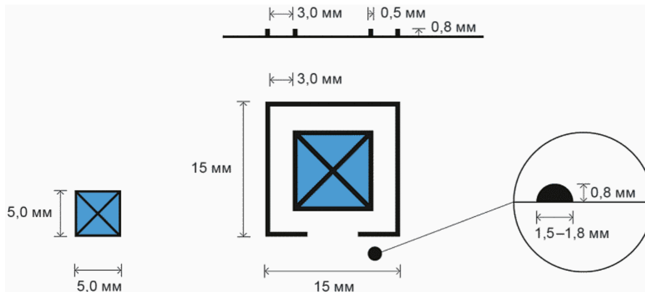
Рисунок 41 - Обозначение лифта на тактильно-визуальной схеме
