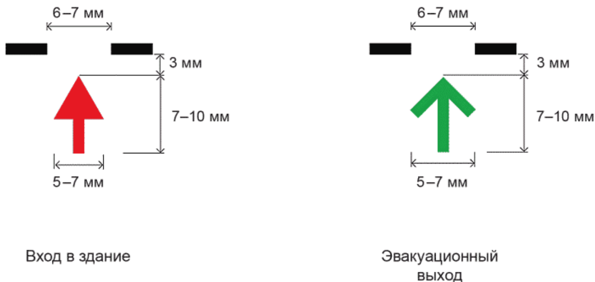
Рисунок 29 - Обозначение входов на объект и эвакуационных выходов
