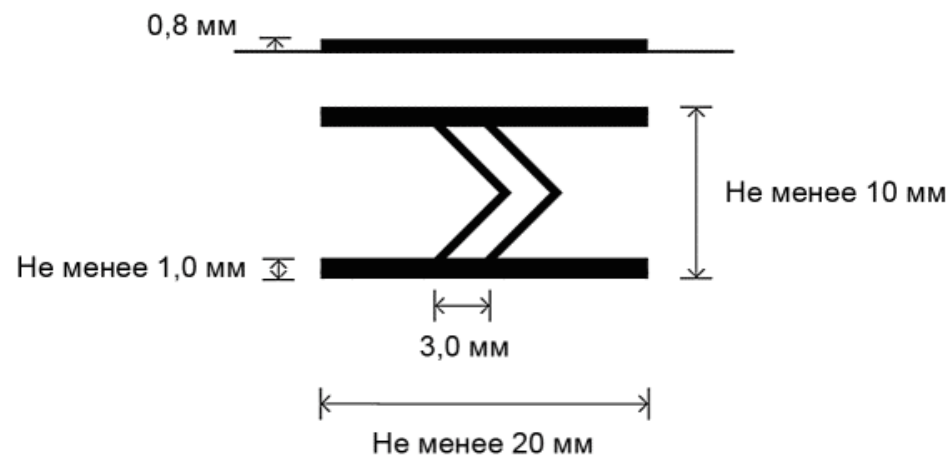
Рисунок 39 - Траволаторы, движущиеся дорожки
