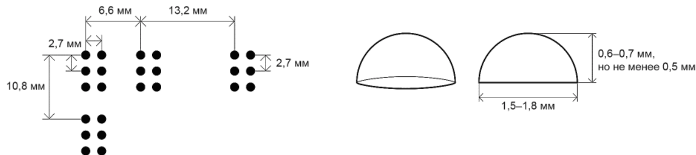
Рисунок 7 - Параметры РТШ
