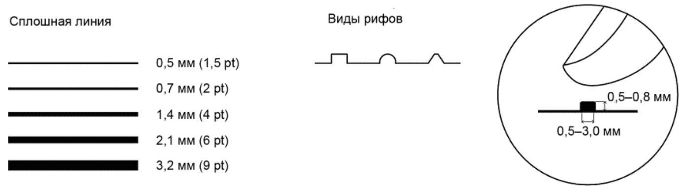
Рисунок 17 - Сплошная линия
