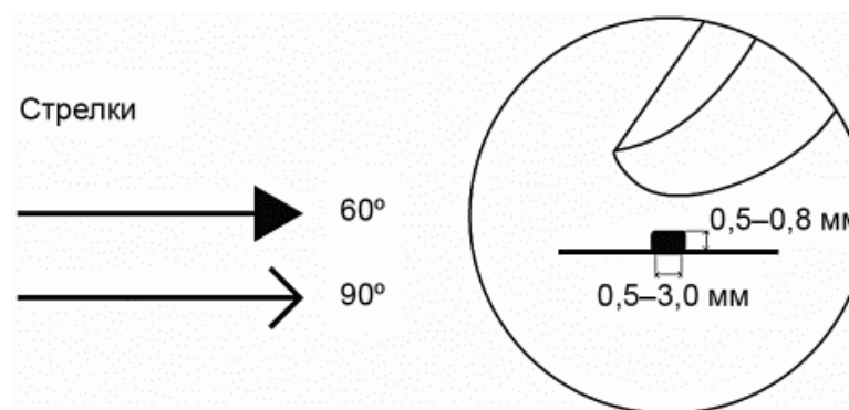
Рисунок 19 - Виды стрелок
