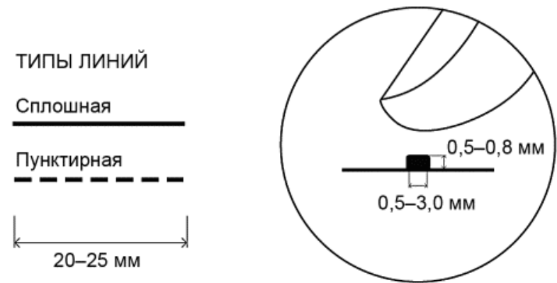
Рисунок 16 - Типы линий
