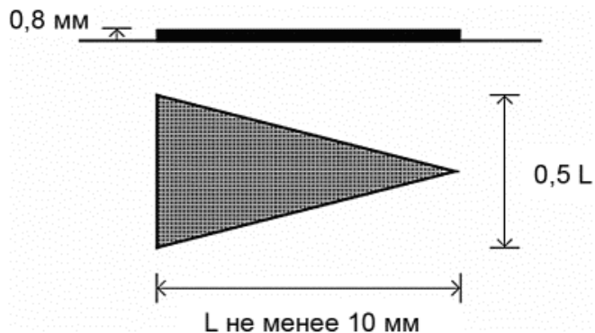
Рисунок 40 - Обозначение марша пандуса
