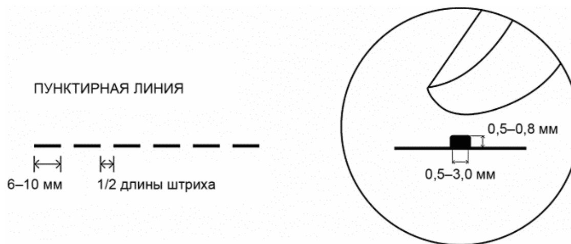
Рисунок 18 - Пунктирная линия
