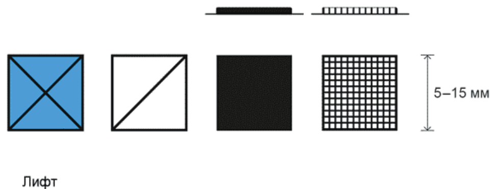
Рисунок 20 - Примеры квадратных рельефных символов
