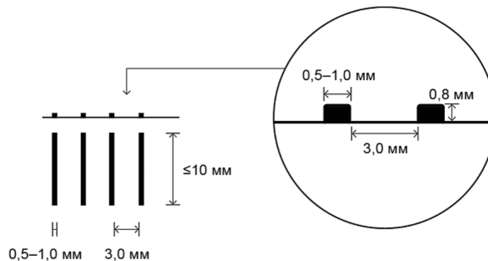
Рисунок 37 - Лестницы
