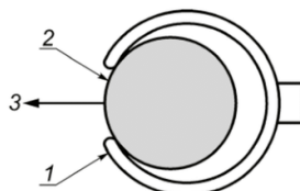
1 — манжета; 2 — цилиндр; 3 — сила растяжения
