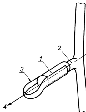
1 — рукоятка; 2 — ручка; 3 — петля из тесьмы; 4 — осевая нагрузка
