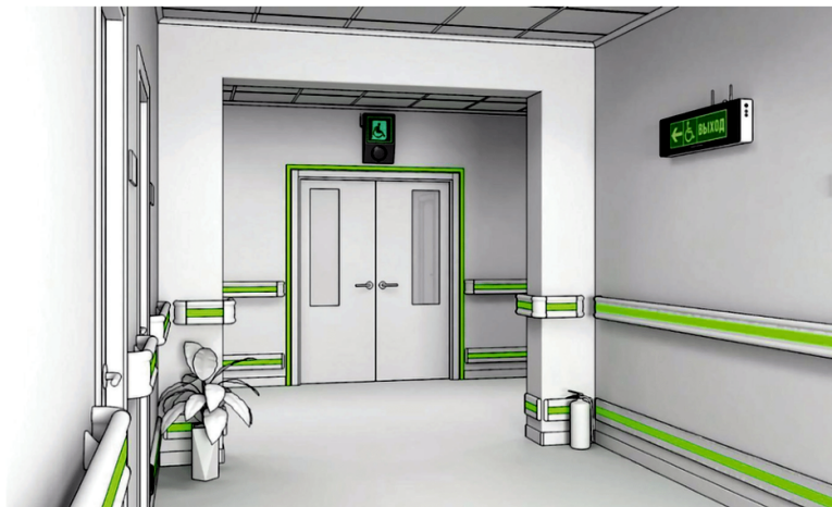
Рисунок А.3 — Пример размещения на стене информационного (визуально-акустического) табло для указания направления движения к эвакуационному выходу, доступному для МГН, в том числе на креслах-колясках
