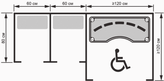
Рисунок 1 — Многосекционная кабина
