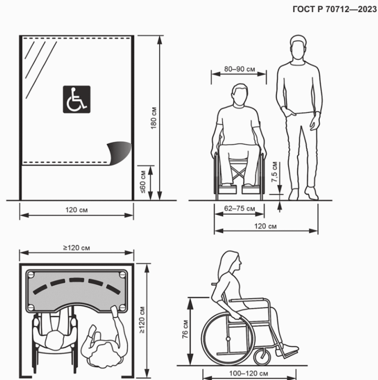
Рисунок 2 — Универсальная кабина и специальная кабина для тайного голосования избирателей, участников референдума, пользующихся креслами-колясками
