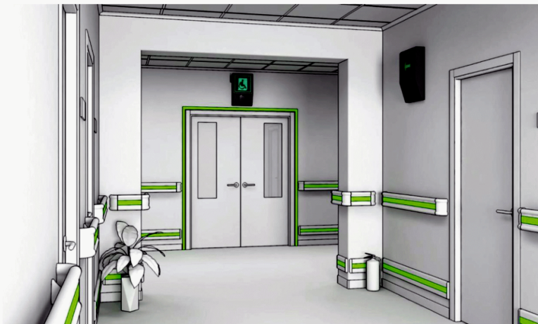
Рисунок А.3 — Пример размещения на стене и над дверью светозвуковых маяков для указания эвакуационного выхода и направления движения к нему, доступному для МГН, в том числе на креслах-колясках
