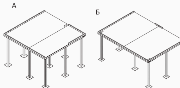
А — горизонтальная секция поворотная на 90°; Б — горизонтальная секция разворотная на 180°
