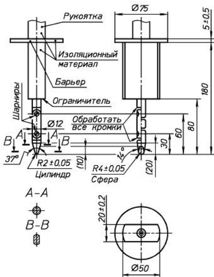
Рисунок 1 - Испытательный шарнирный палец
