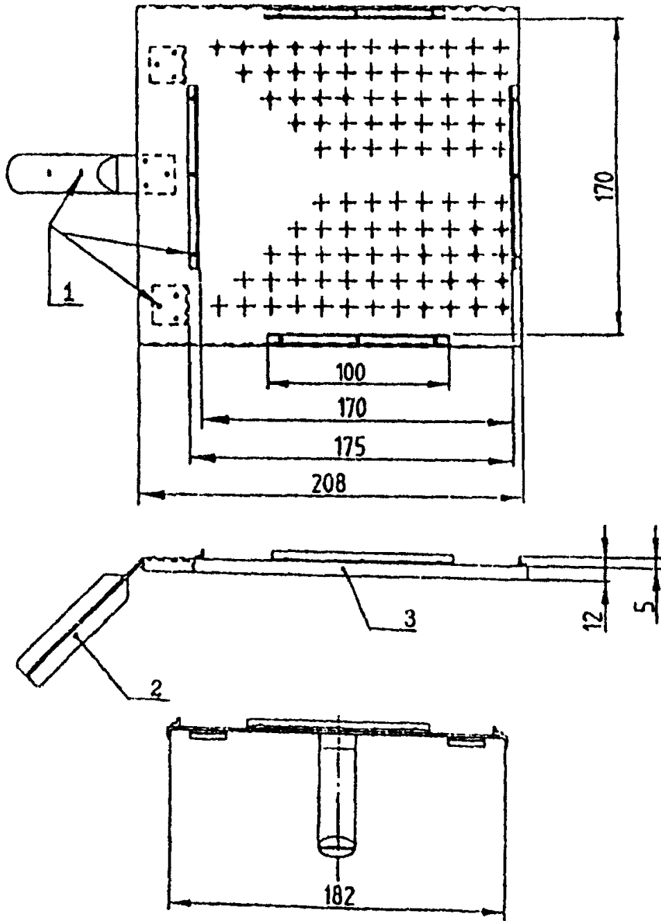
1 - заклепки; 2 - рукоятка;
