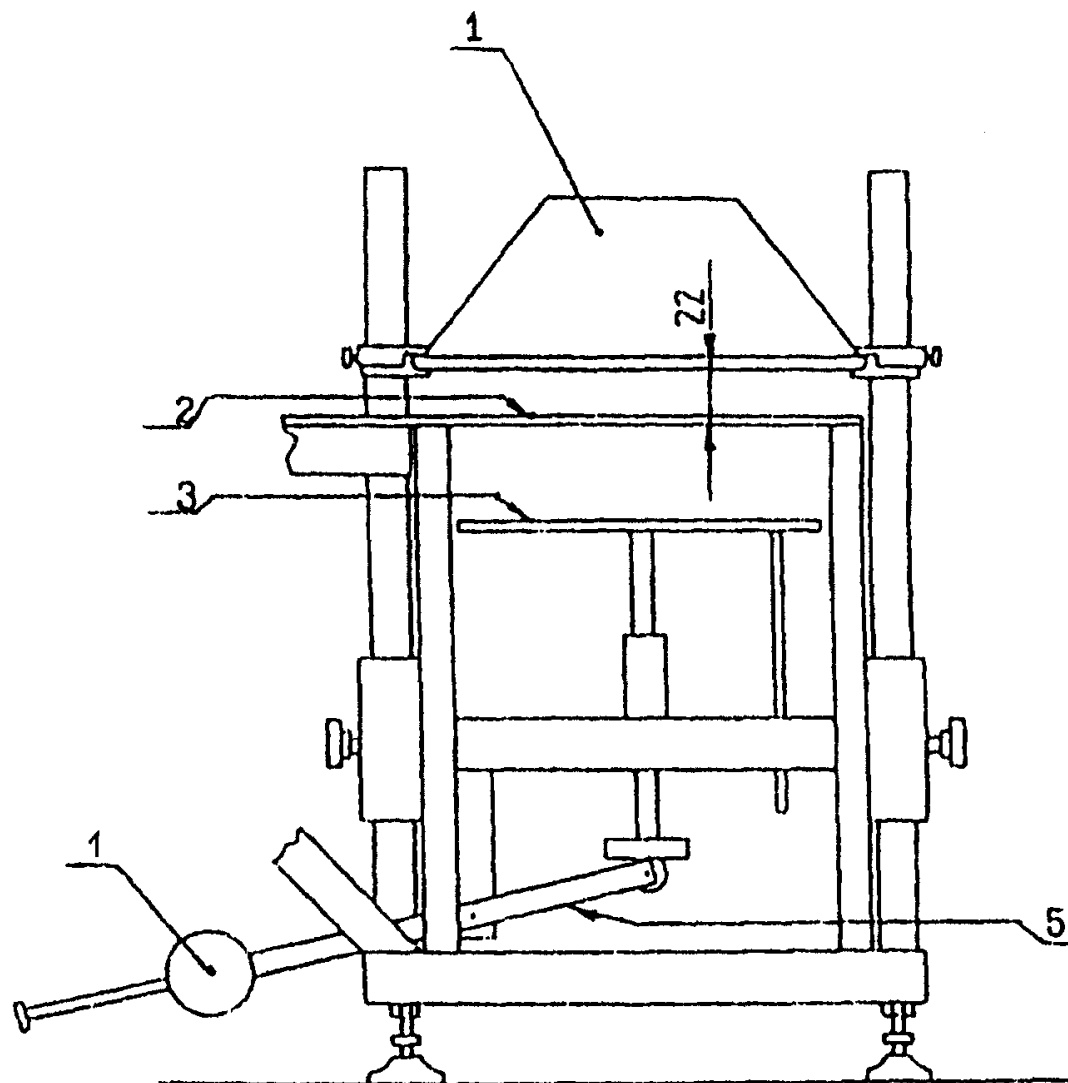
Рисунок А3. Опорная станина (разрез по АА)
