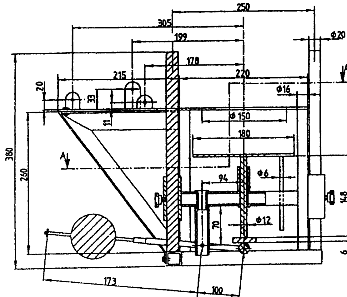
Рисунок А2. Опорная станина (разрез по ВВ)
