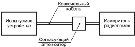
Рисунок 9 — Структурная схема измерения напряжения радиопомех и полезного сигнала на ВЧ-выходе испытуемого устройства
