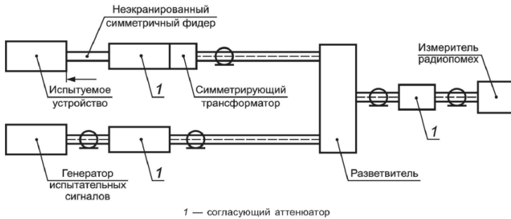
1 — согласующий аттенуатор Рисунок 8 — Структурная схема измерения напряжения ИРП на симметричном антенном входе
