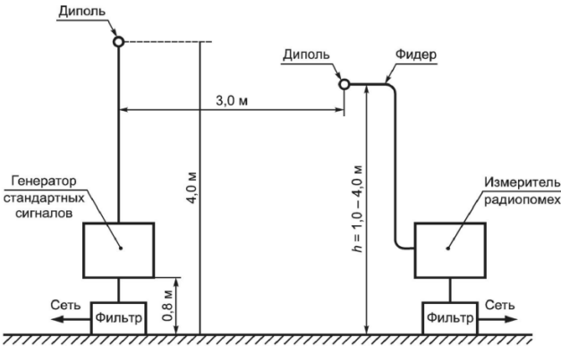
Рисунок 12 — Расположение аппаратуры при аттестации площадки
