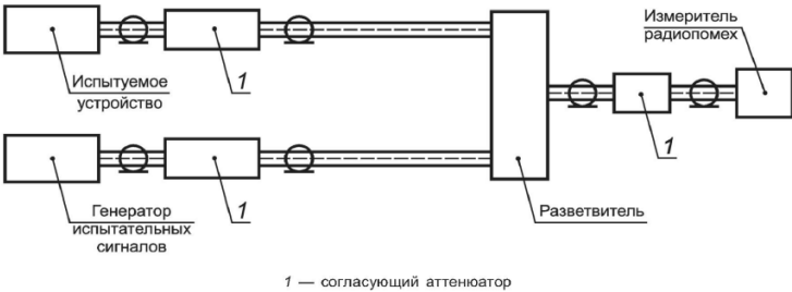
1 — согласующий аттенуатор Рисунок 7 — Структурная схема измерения напряжения ИРП на коаксиальном антенном входе
