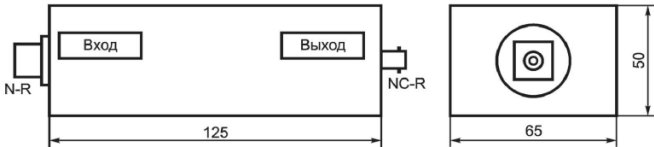
Рисунок А.3 — Типовые размеры развязывающего трансформатора с рабочей полосой частот от 46 МГц до 1,5 ГГц
