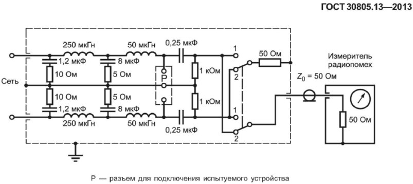
Рисунок 4 — Пример схемы v-образного эквивалента сети 50 Ом/50 мкГн + 5 Ом
