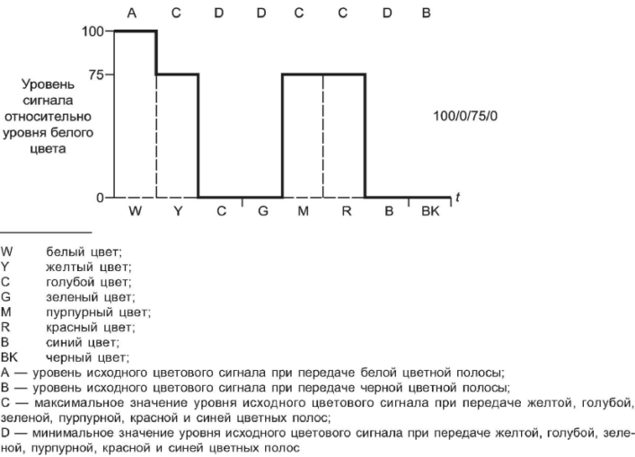
Рисунок 1 — Уровни сигналов цветных полос (сигнал красного цвета) номенклатуры 100/0/75/0 (ГОСТ 9021)
