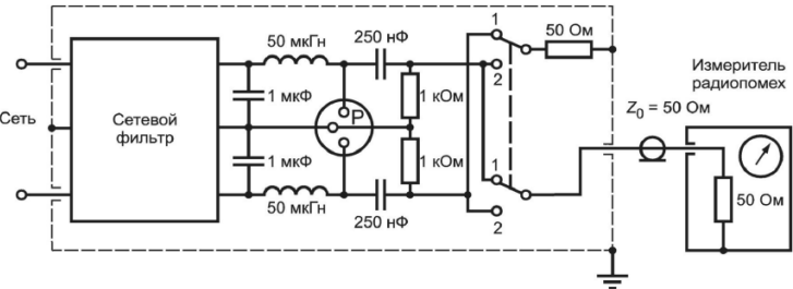
Рисунок 3 — Пример схемы V-образного эквивалента сети 50 Ом/50 мкГн
