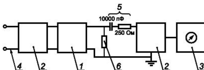
Рисунок 5 - Схема измерения ИРП от регулирующих устройств
