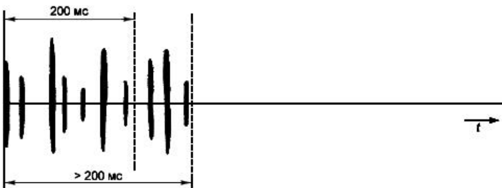
Рисунок 3 - Примеры прерывистых ИРП, нормируемых как кратковременные
