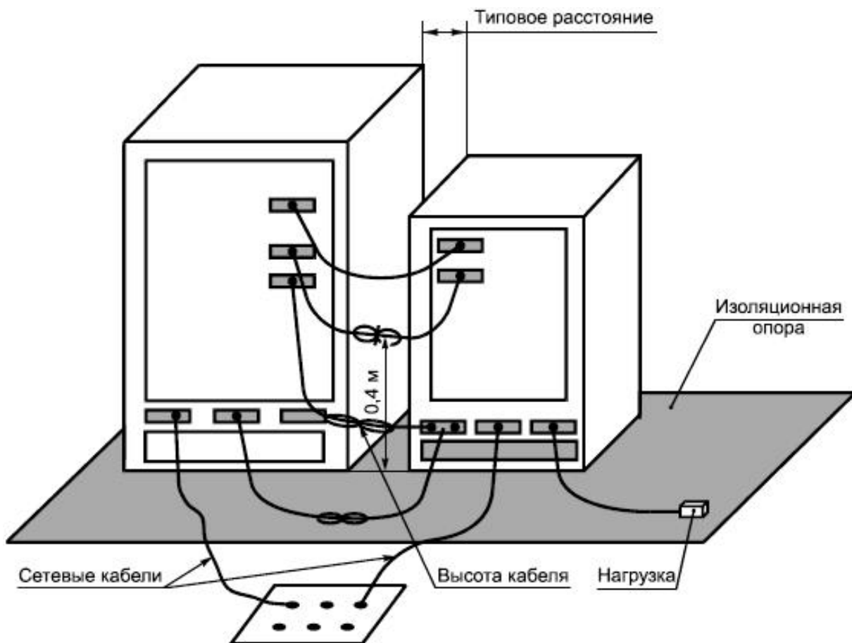
Рисунок 11 - Размещение ИО: напольное оборудование, измерение излучаемых ИРП
