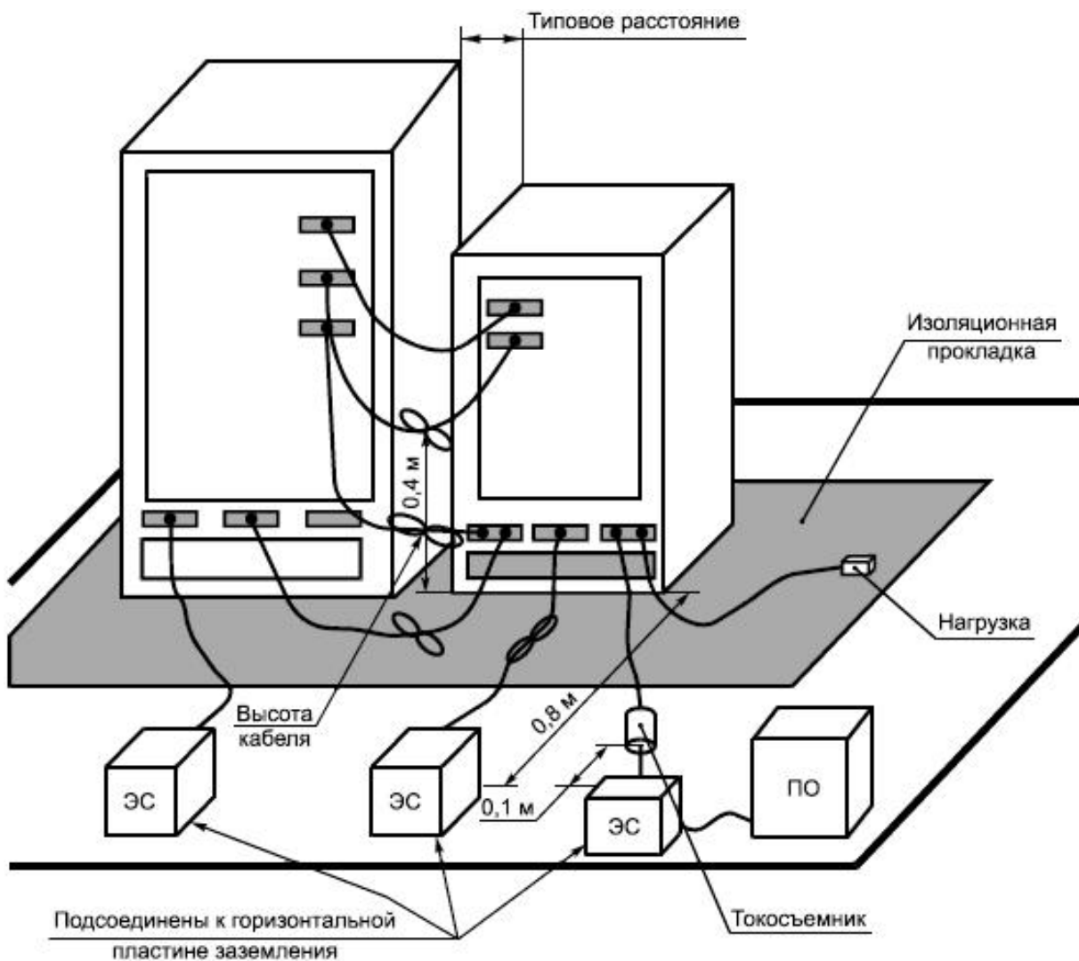
Рисунок 8 - Размещение ИО: напольное оборудование, измерение кондуктивных ИРП
