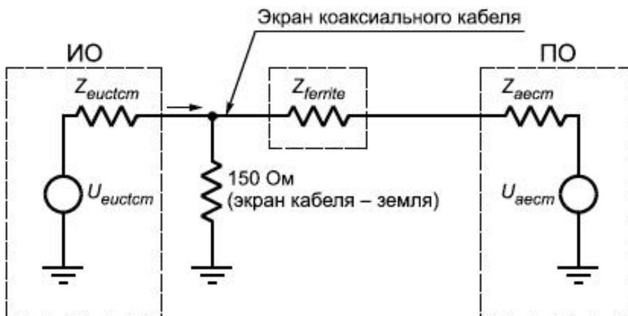
Рисунок Ф.3 - Полные сопротивления элементов (см. рисунок С.2)
