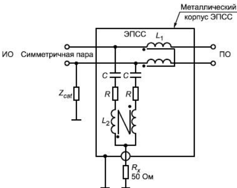
Рисунок D.1 - ЭПСС для применения с одной неэкранированной симметричной парой
