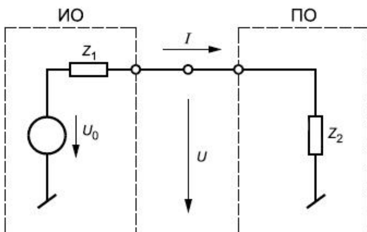
Рисунок F.2 - Основная схема проведения измерений при неизвестном общем несимметричном полном сопротивлении
