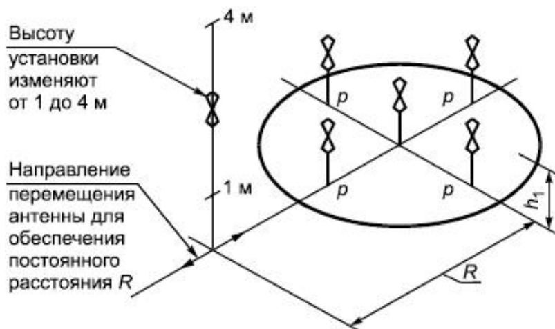
Рисунок А.1 - Типичное расположение антенн при измерении затухания альтернативной измерительной площадки
