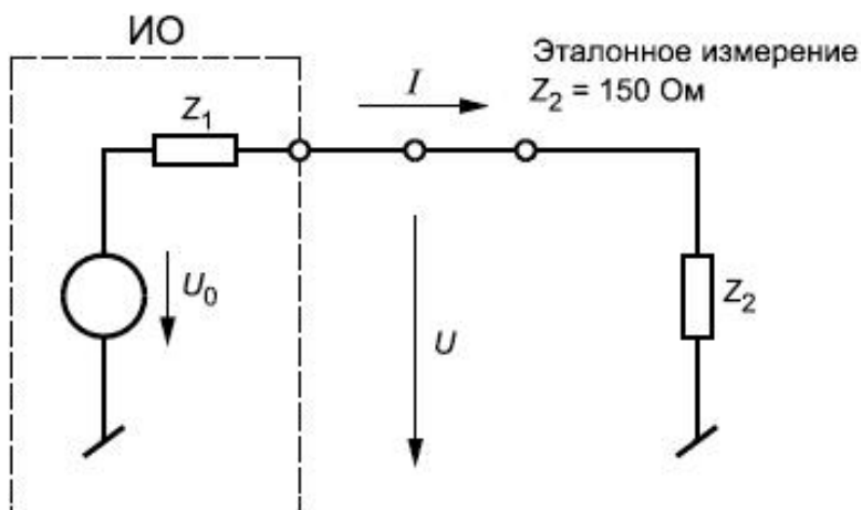
Рисунок F.1 - Основная схема рассмотрения норм при заданном значении общего несимметричного полного сопротивления, равном 150 Ом
