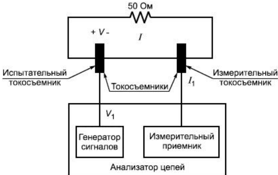
Рисунок С.5 - Установка для калибровки
