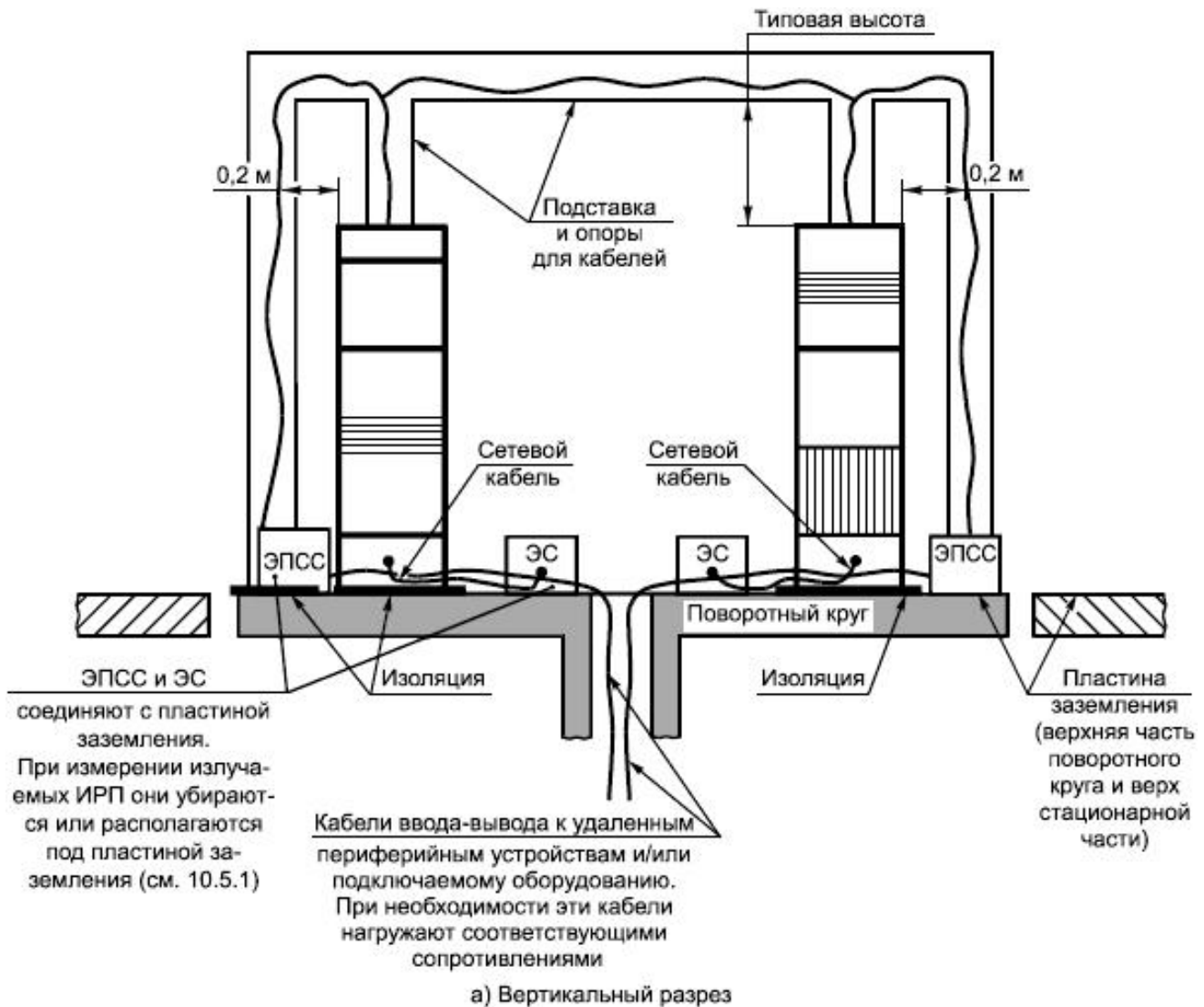
Рисунок 12 - Размещение ИО: напольное оборудование с вертикальными стойками и воздушными кабелями, измерение кондуктивных и излучаемых ИРП
