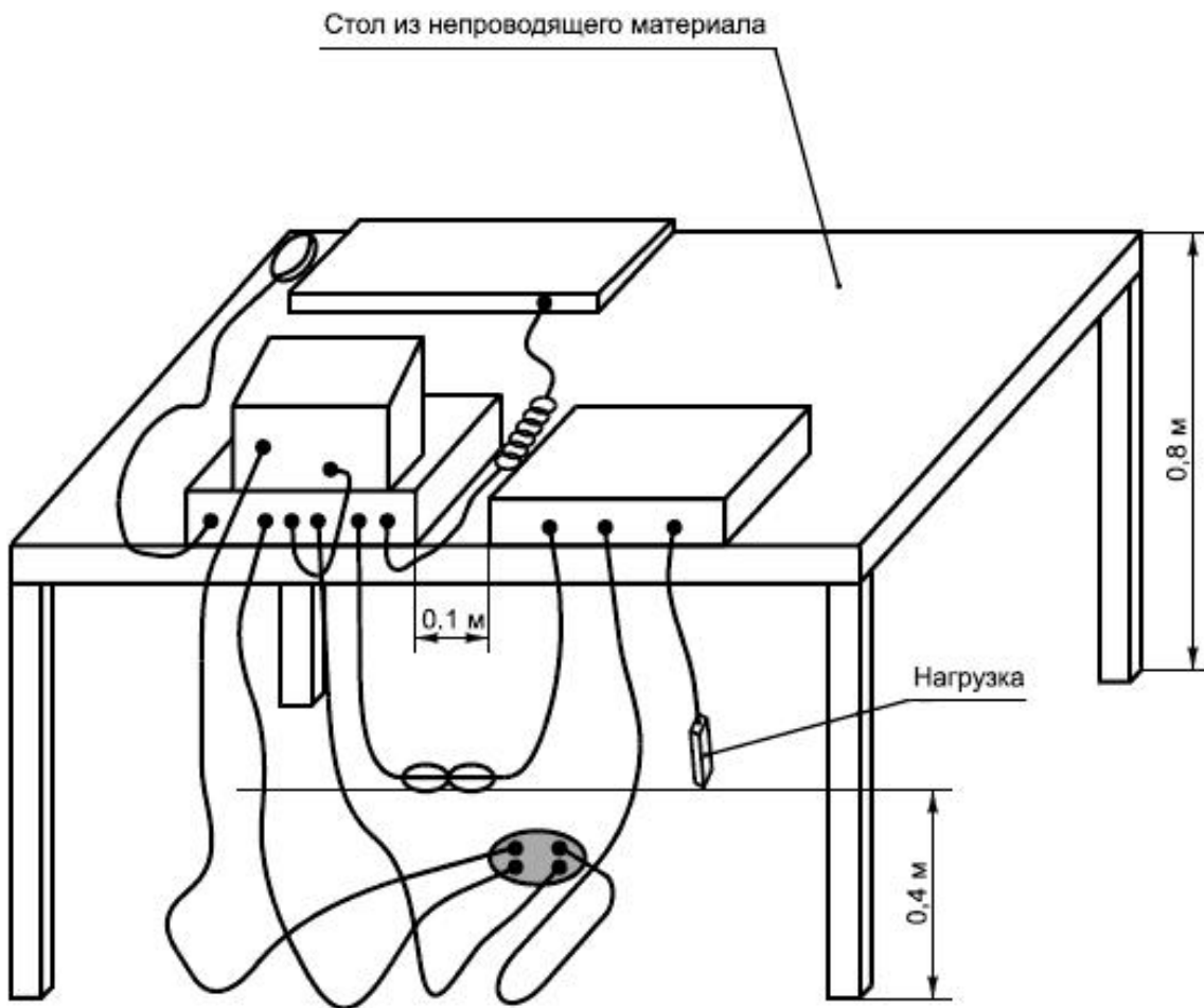
Рисунок 10 - Размещение ИО: настольное оборудование, измерение излучаемых ИРП
