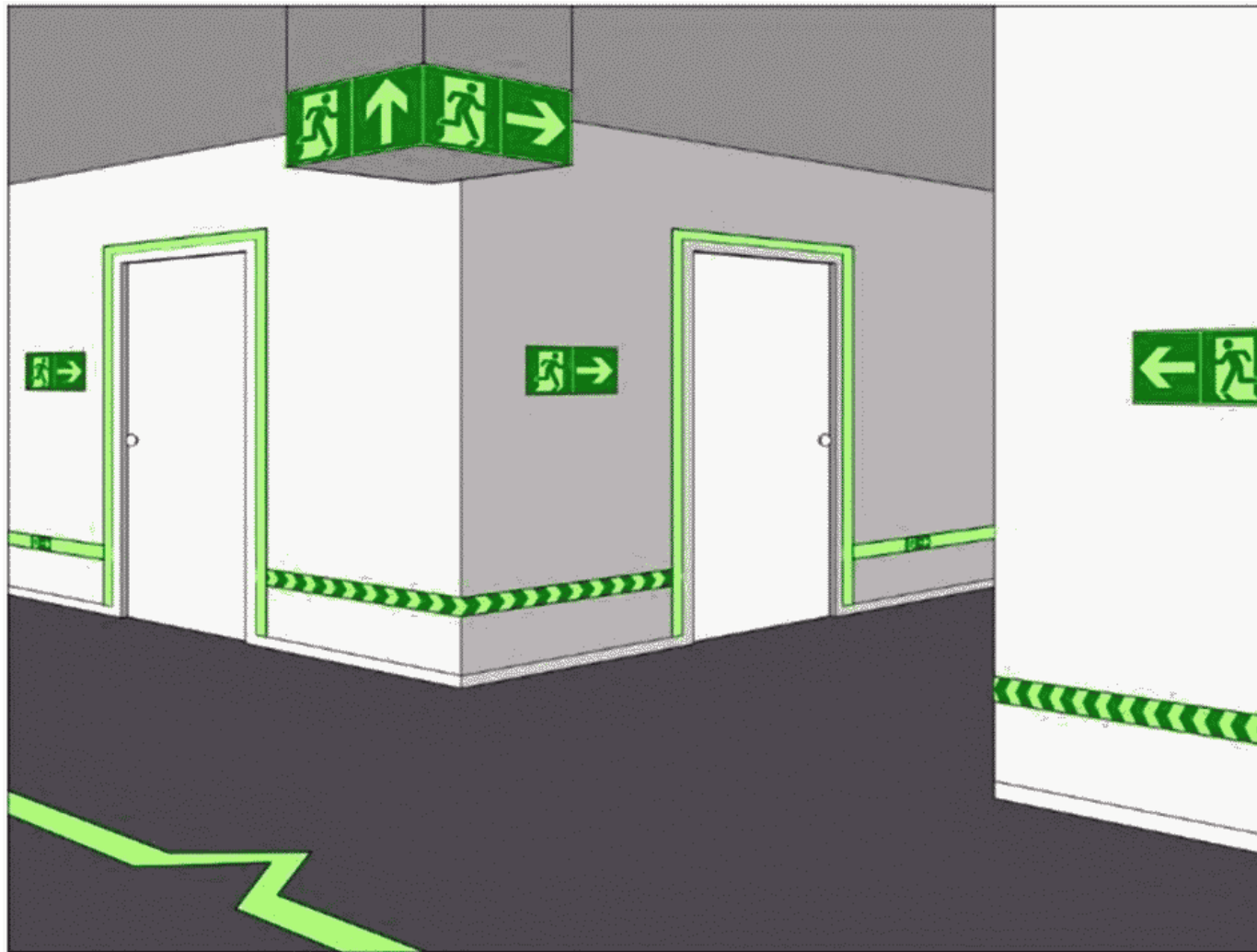
Рисунок В.11 - Пример комбинированного обозначения эвакуационного пути в широких коридорах, проходных помещениях и т.п.
