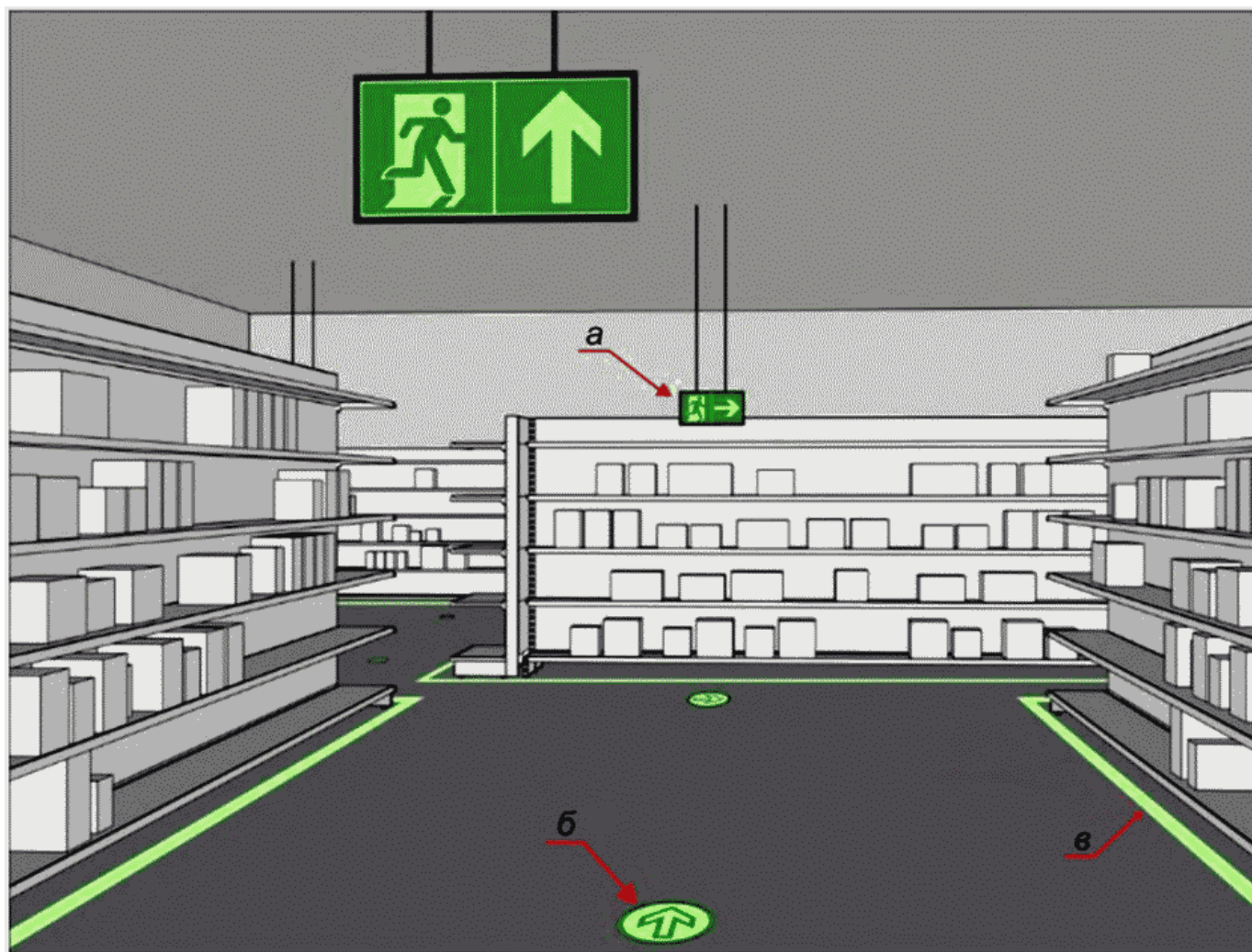
a - потолочный комбинированный указатель направления эвакуации; б - напольный основной указатель направления эвакуации; в - напольная направляющая линия
