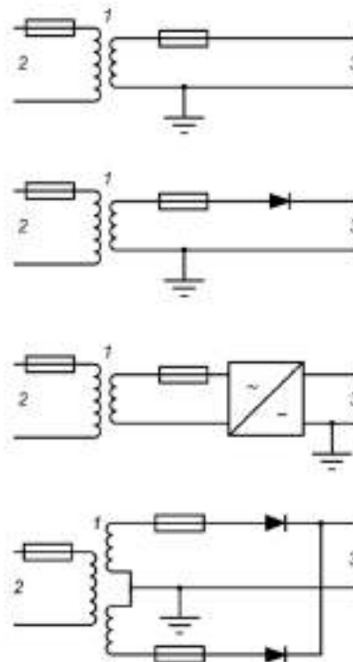
Рисунок 3 — Питание цепей управления
