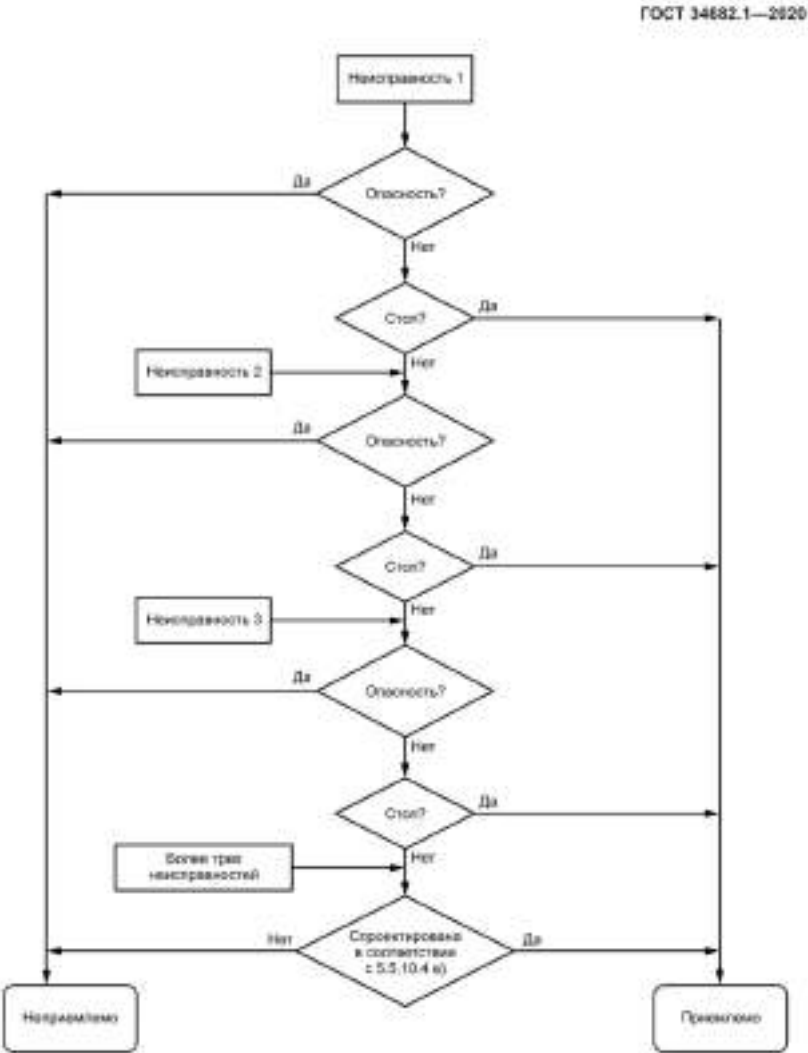
Рисунок 5 — Схема оценки цепи безопасности
