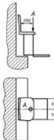
Рисунок 2 — Грузонесущие устройства для перевозки пользователя в положении сидя
