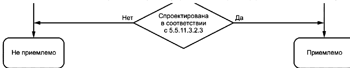
Рисунок 5 - Блок-схема оценки цепи безопасности
