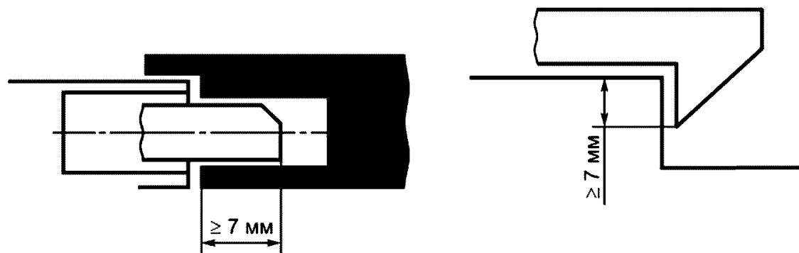
Рисунок 10 - Пример запирающего элемента
