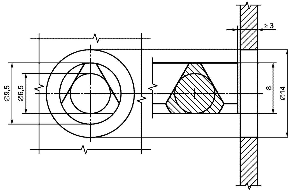
Рисунок 11 - Треугольная ключевина
