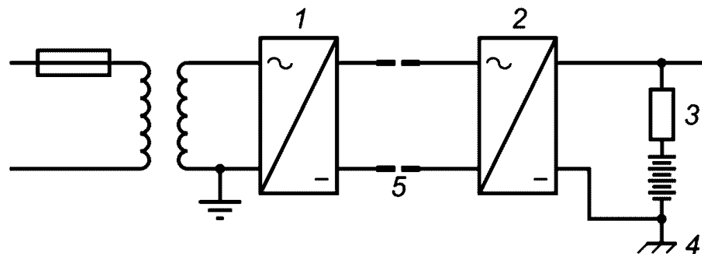
b) Зарядное устройство постоянного тока AD
