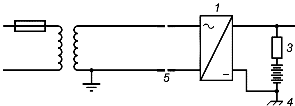
а) Зарядное устройство переменного тока AC
