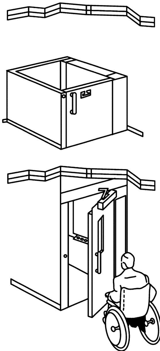
Рисунок 7 — Пример вертикальной платформы с огражденной шахтой
