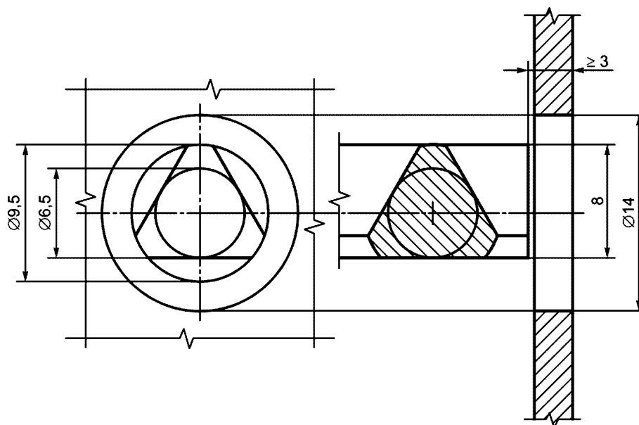
Рисунок 11 — Треугольная ключевина
