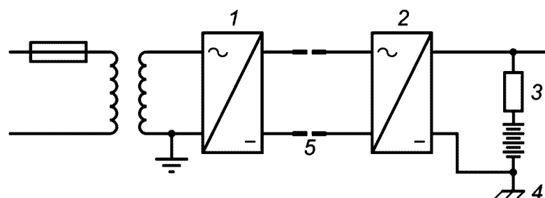
б) Зарядное устройство постоянного тока AD
