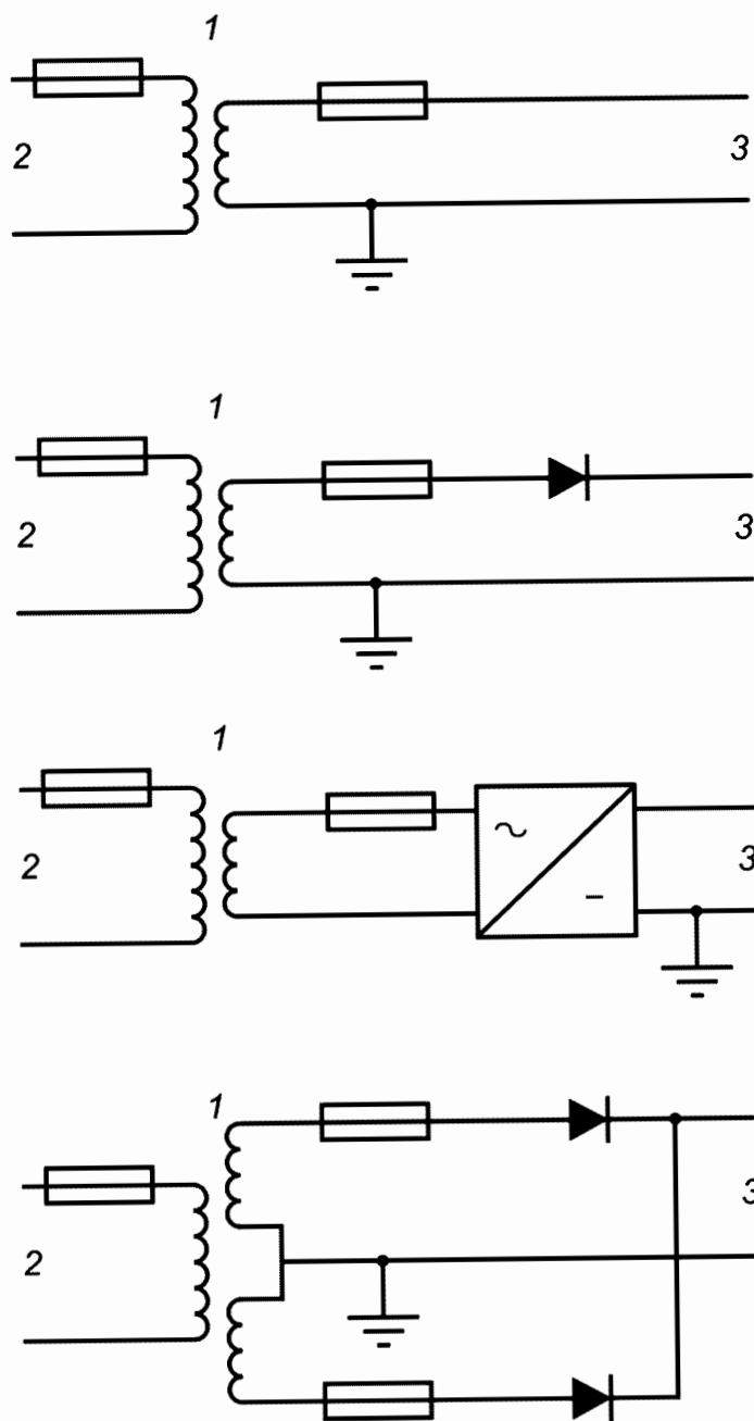
1 — разделительный трансформатор; 2 — первичный источник; 3 — схема управления
