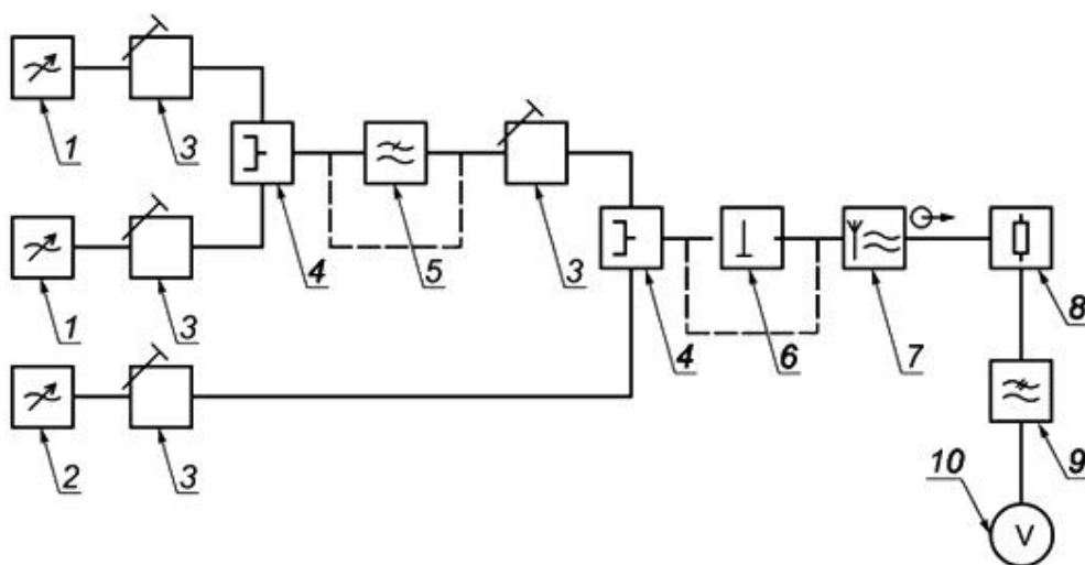
Рисунок 4 - Структурная схема установки для измерения помехоустойчивости по входу телевизионных приемников и магнитофонов
