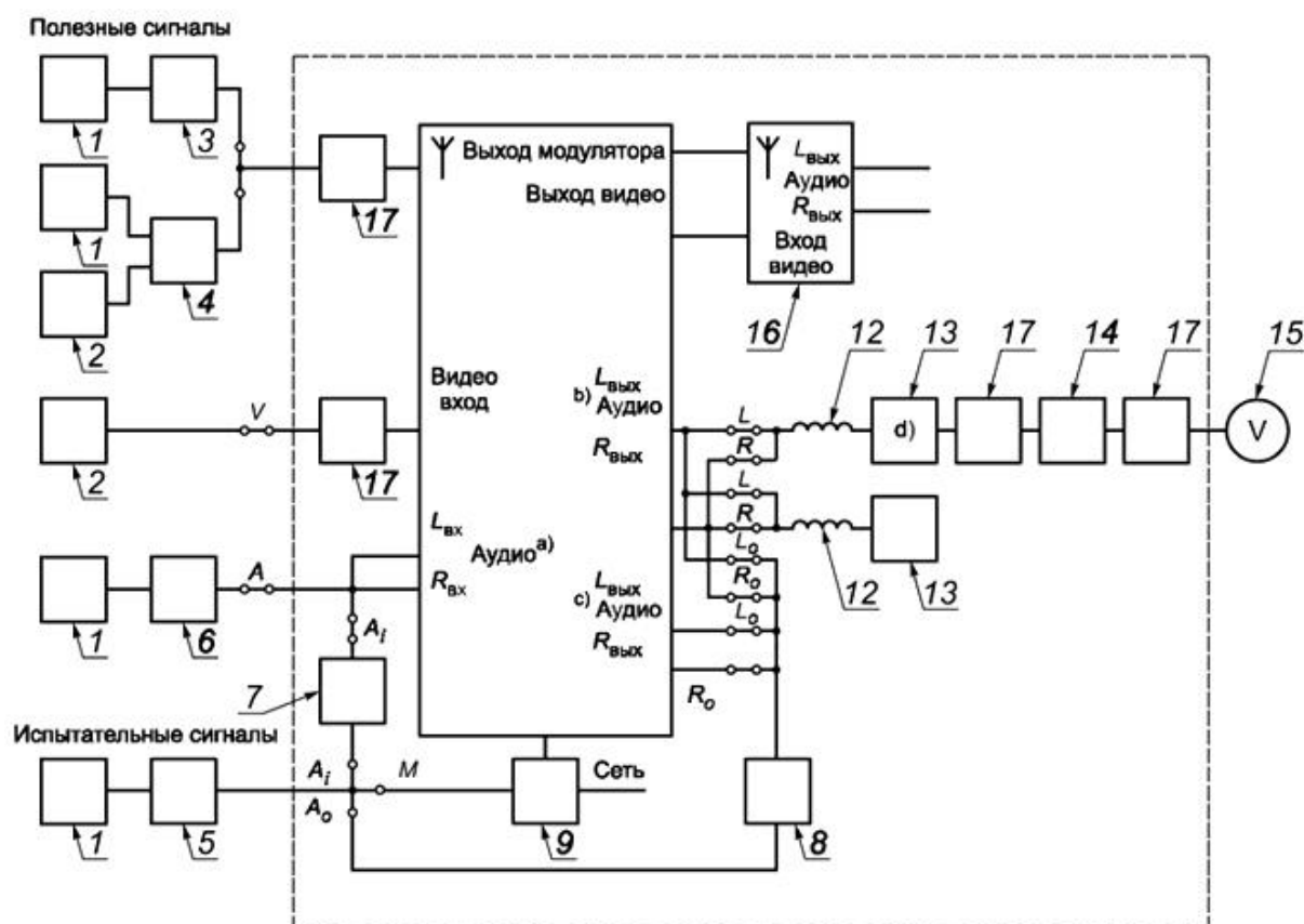
Рисунок 8 - Структурная схема измерения устойчивости к наведенным напряжениям на сетевом входе, выходе наушников, громкоговорителей, звуковом выходе, звуковом входе
