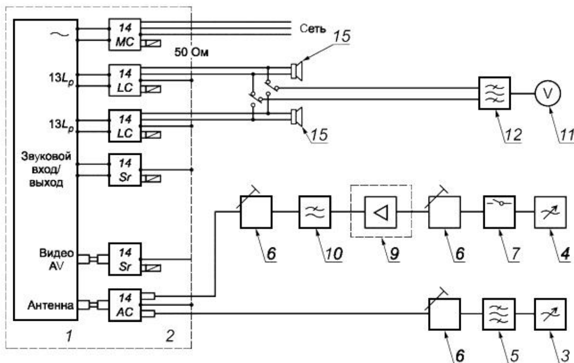
Рисунок 6 - Структурная схема измерения устойчивости к наведенным токам
