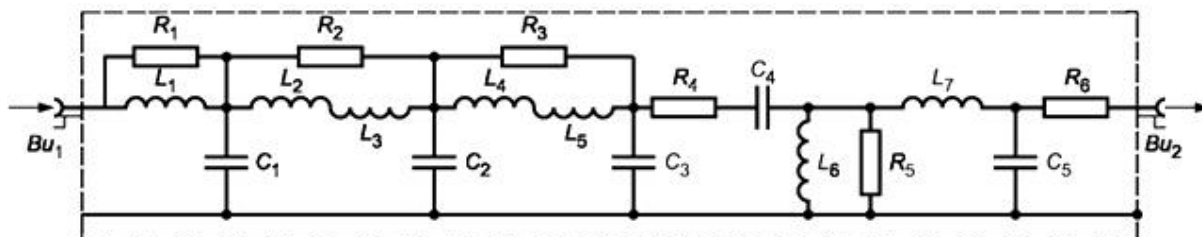
Рисунок В.1 - Полосовой фильтр 0,5-3 кГц
