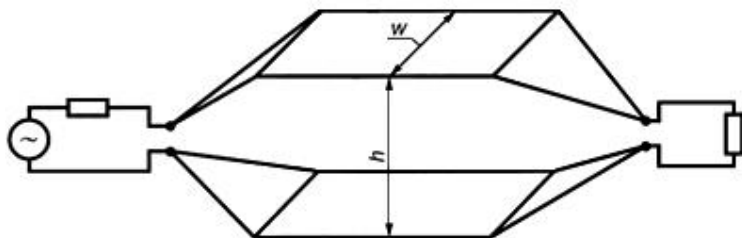
Рисунок Е.1 - ТЕМ-устройство на открытой полосковой линии; базовая конфигурация с согласующей схемой и нагрузкой
