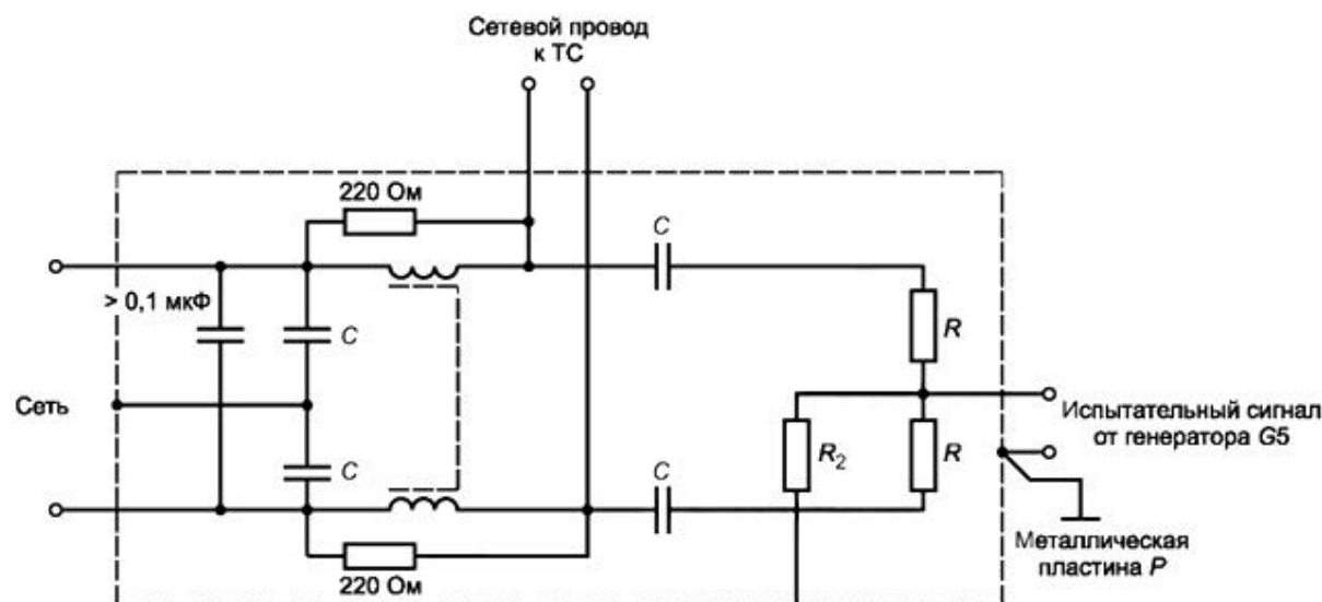
Рисунок D.3 - Сетевой режекторный фильтр MSF
