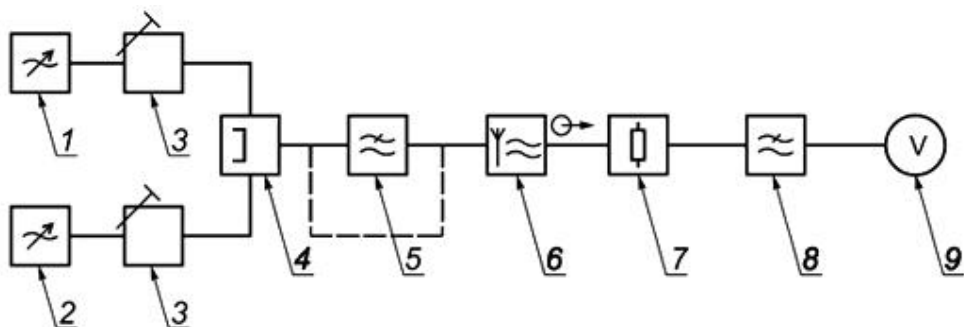
Рисунок 3 - Структурная схема измерения помехоустойчивости по входу звуковых приемников
