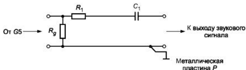
Рисунок D.2 - Цепь RC для выходов звукового сигнала RC(o)
