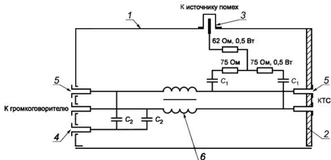
Рисунок С.3 - Конструкция блока УСР типа LC (для проводов громкоговорителя)
