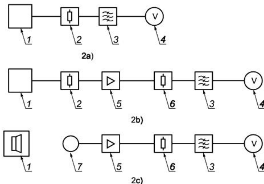
Рисунок 2 - Структурная схема измерения выходной мощности звукового сигнала
