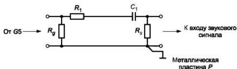
Рисунок D.1 - Цепь RC для входов звукового сигнала RS(i)
