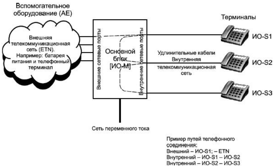
Рисунок А.5 - Пример типовой микро-АТС или мини-АТС
