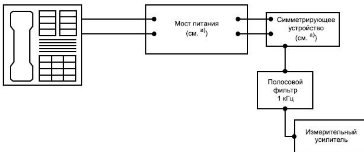
Рисунок А.4 - Установка для измерения демодуляции в аналоговых линиях
