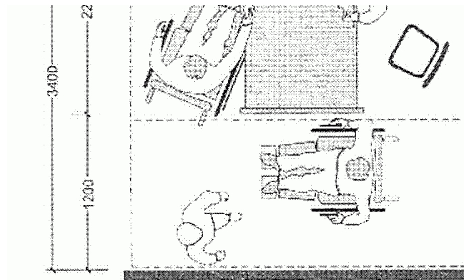
Рисунок Б.13 - Зоны обслуживания и зоны проезда в палатах для лежачих больных
