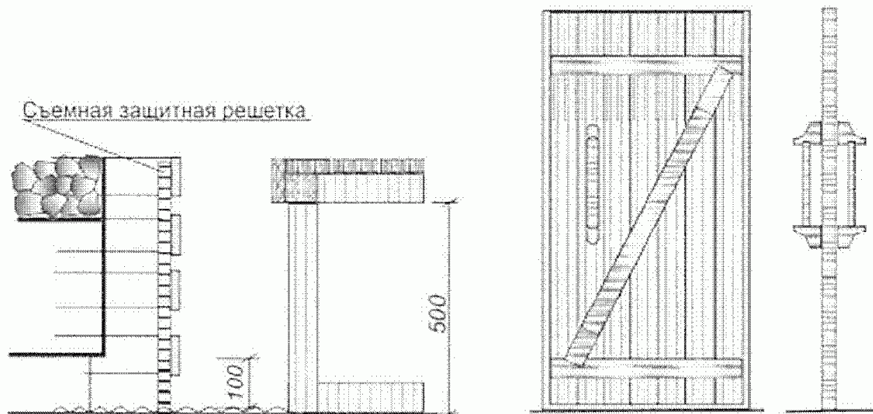
Рисунок Б.25 - Оборудование сауны
