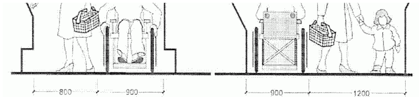
Рисунок Б.14 - Оборудование предприятий торговли
