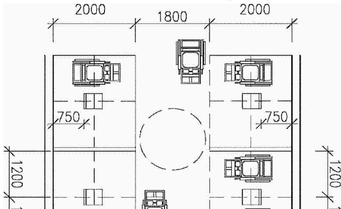
Рисунок Г.2 - Зона расположения инвалидных колясок
