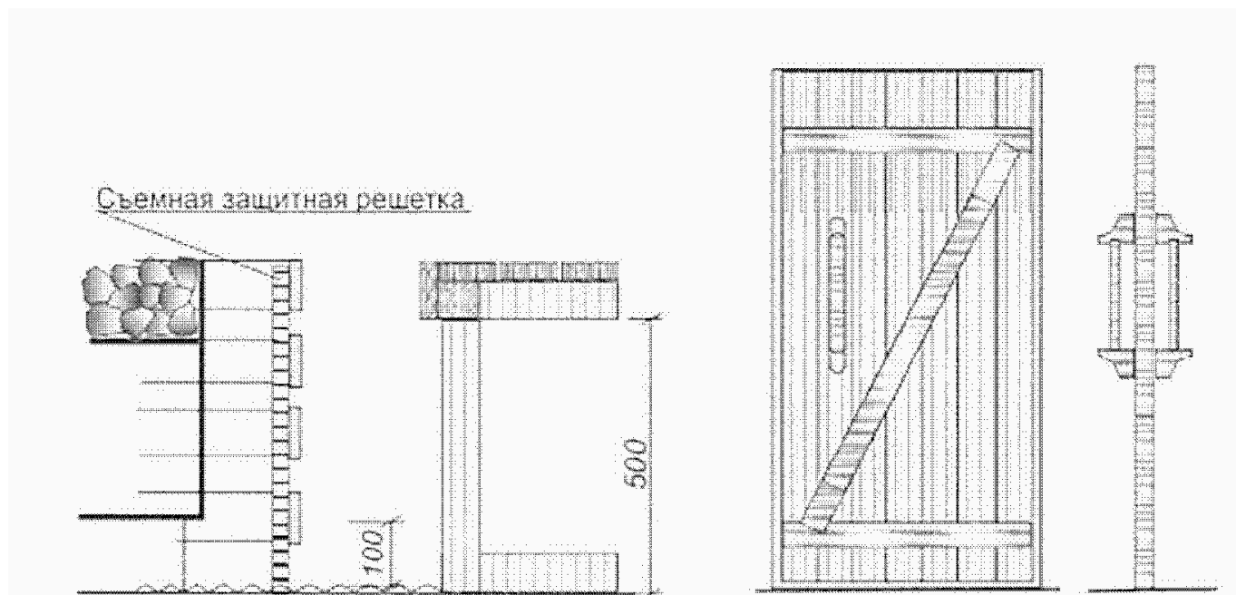
Рисунок Б.25 - Оборудование сауны
