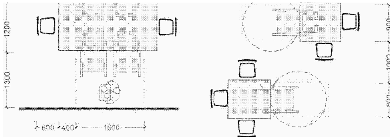
Рисунок Б.19 - Примеры размещения мест в залах предприятий общественного питания
