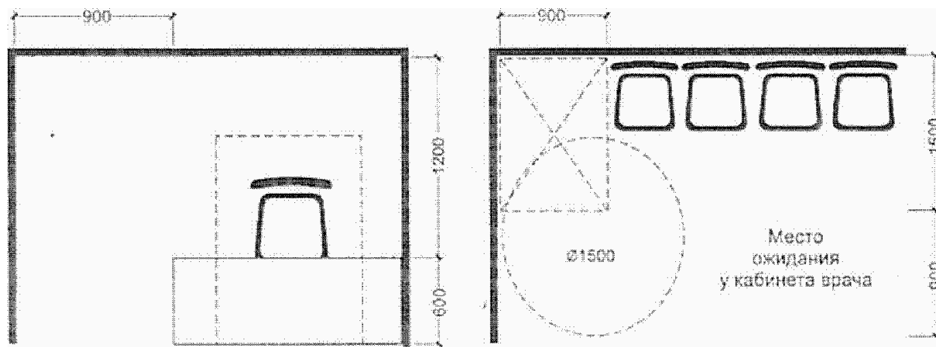
Рисунок Б.8 - Примеры расстановки оборудования
