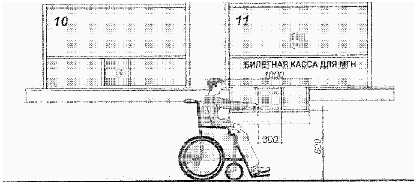
Рисунок Б.21 - Оборудование вокзалов
