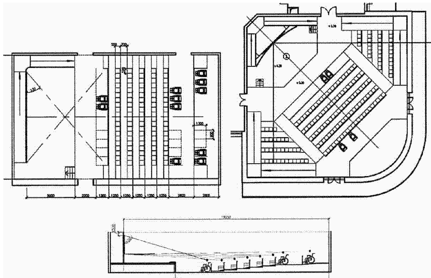
Рисунок Г.8 - Варианты планировочного решения зрительного зала
