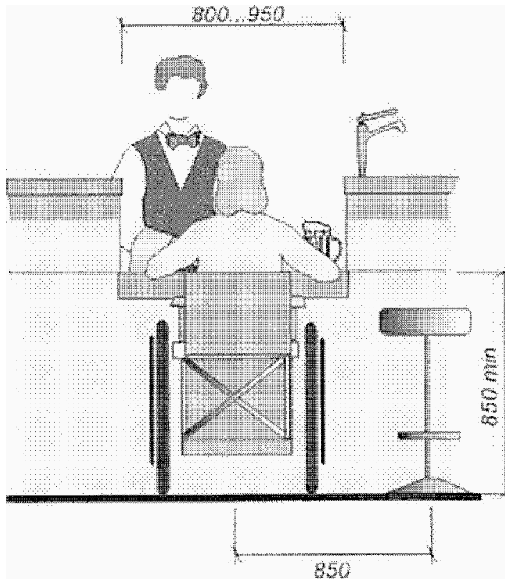
Рисунок Б.16 - Оборудование предприятий питания
