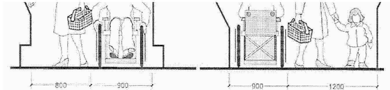
Рисунок Б.14 - Оборудование предприятий торговли
