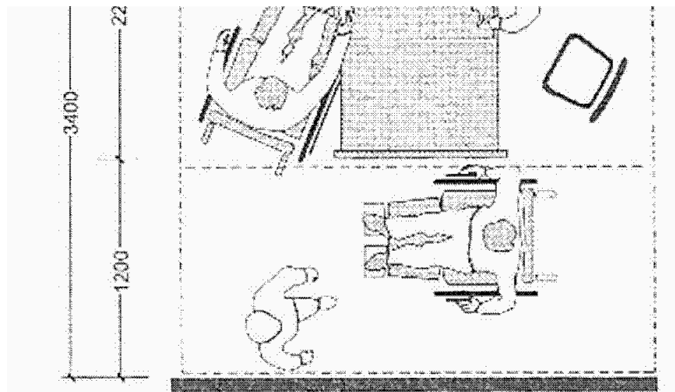
Рисунок Б.13 - Зоны обслуживания и зоны проезда в палатах для лежащих больных
