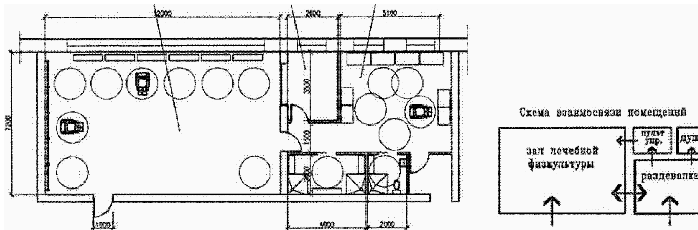
Рисунок Г.7 - Зал лечебной физкультуры
