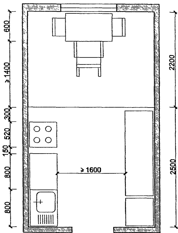
ГАБАРИТЫ УСТАНОВКИ ОБОРУДОВАНИЯ
