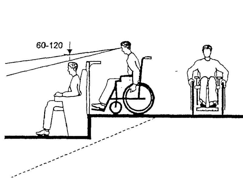
Превышение луча зрения для инвалидов в кресле-коляске
