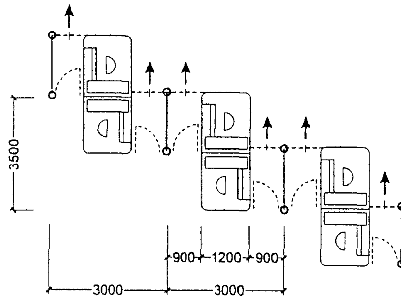
ФРАГМЕНТ ПЛАНА ЗОНЫ ВЫДАЧИ БАГАЖА ПРИ ПОДАЧЕ С НИЖЕЛЕЖАЩЕГО ЭТАЖА
