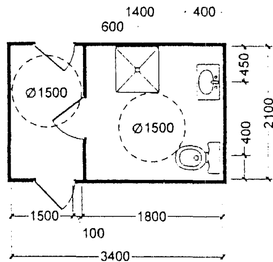
Санитарный узел с прихожей при номере гостиницы
