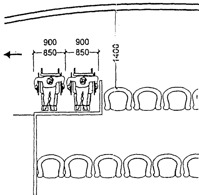
Рис. 6.7. Места для инвалидов в зрительных залах
