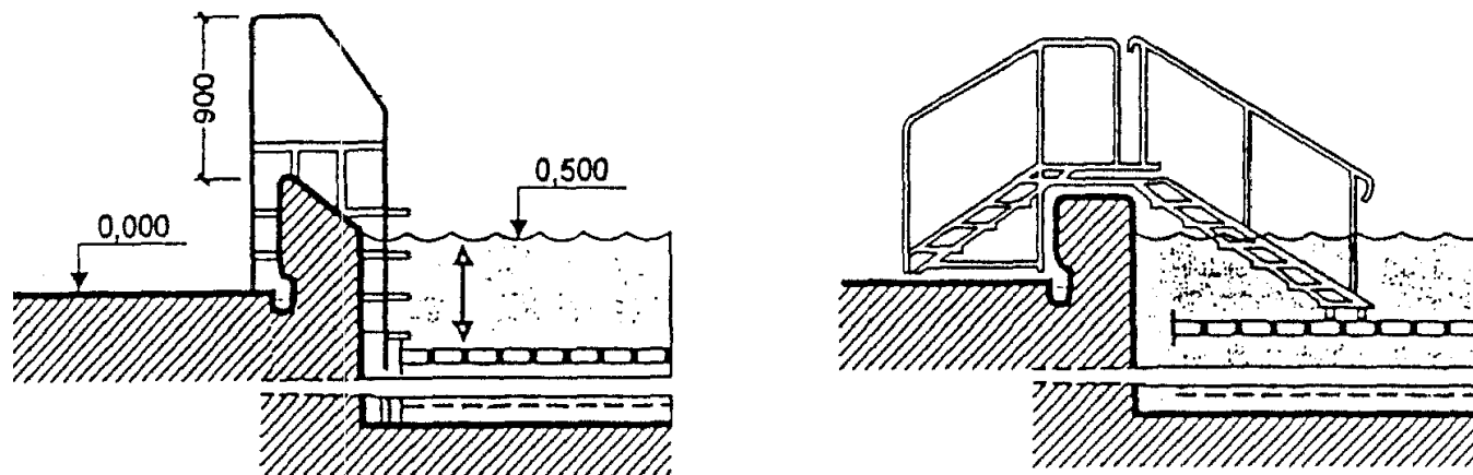
Рис. 5.2. Плавательный бассейн
