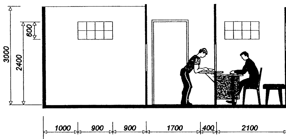
Разрез 1-1
