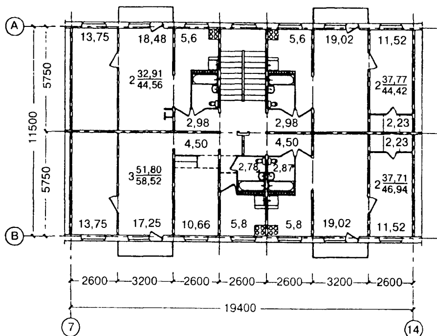
А. Существующее положение План типового этажа рядовой секции 2-2-2-3
