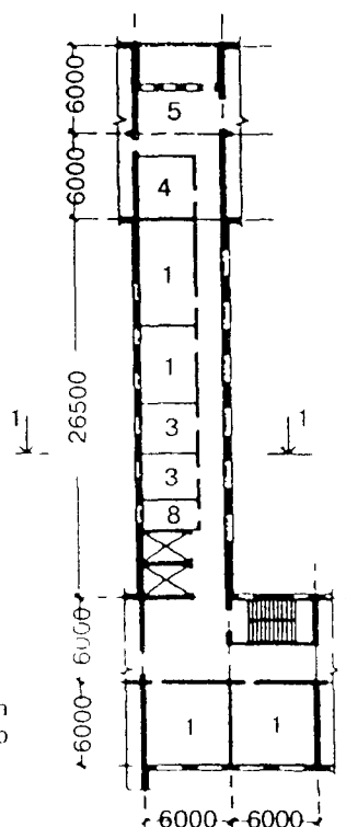
Фрагмент плана 3-го этажа
