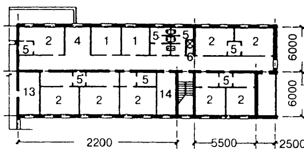
Фрагмент плана 1-го этажа
