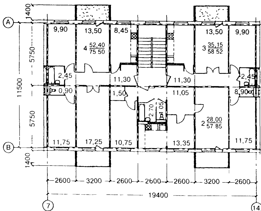
Б. Проектное предложение План типового этажа рядовой секции 2-3-4
