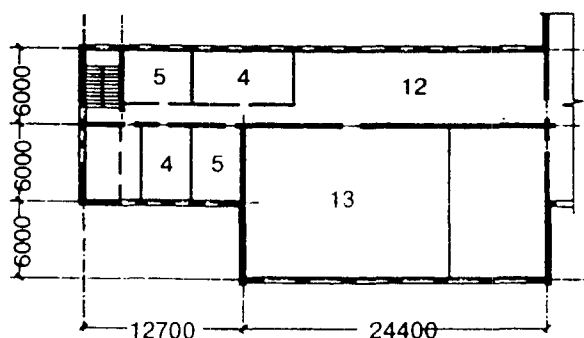
Фрагмент плана 2-го этажа
