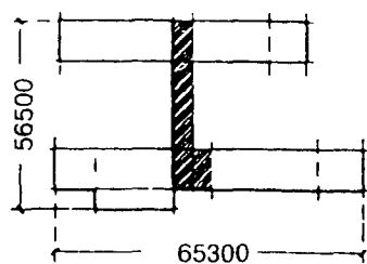
План здания
