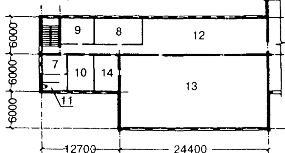
Фрагмент плана 2-го этажа
